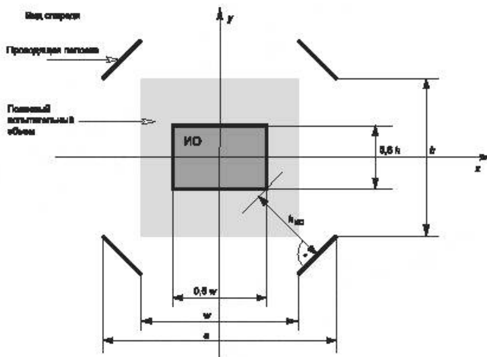
Рисунок А.9б — Поперечное сечение волновода
