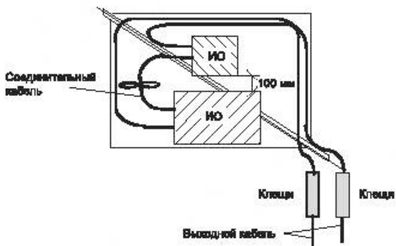
Рисунок А.1b — Вид сверху
