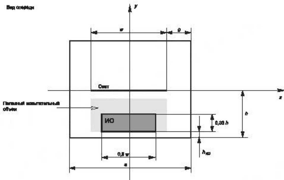
Рисунок А.6b — Поперечное сечение камеры
