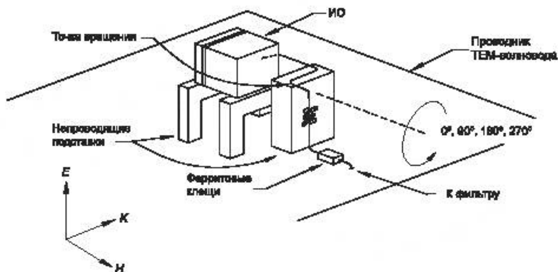
Рисунок В.1а — Положения ИО для вертикальной поляризации
