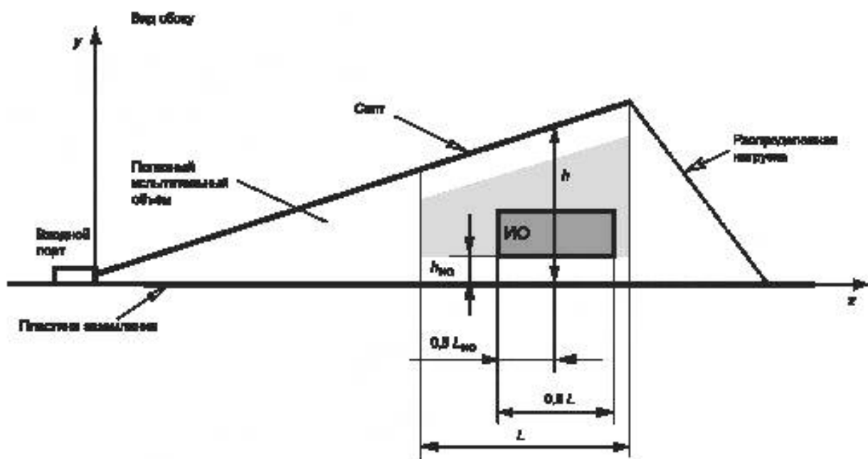
Рисунок A.8a — Вид сбоку (однопортовый волновод)
