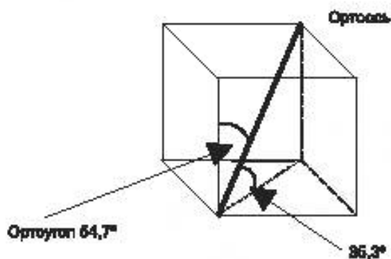
Рисунок А.2а — Ортоось и ортоугол
