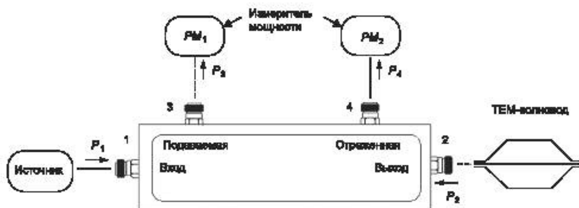
Рисунок Е.3 — Общая схема для измерения подаваемой мощности на передающее устройство
