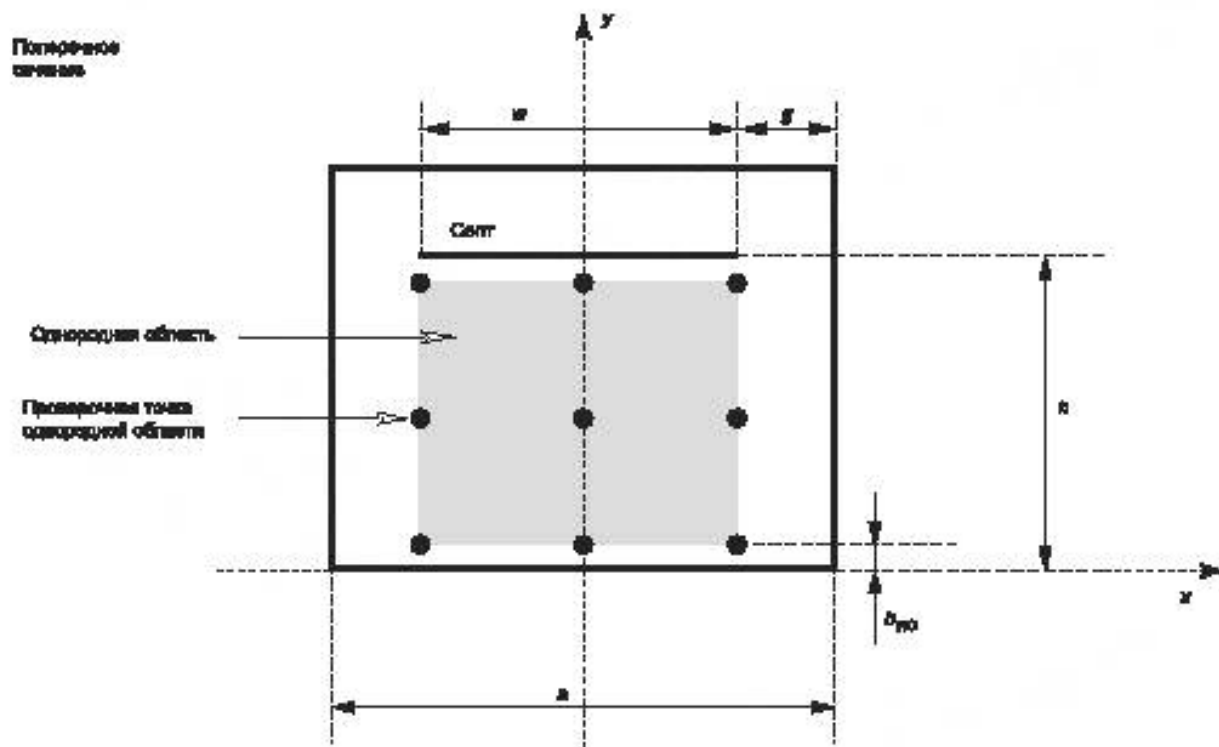
Рисунок В.2b — Поперечное сечение
