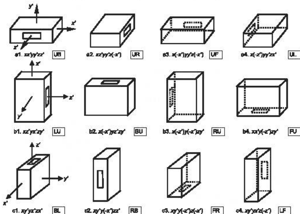
Рисунок A.3 — Три ортогональные оси вращения положений для измерения помехозащиты
