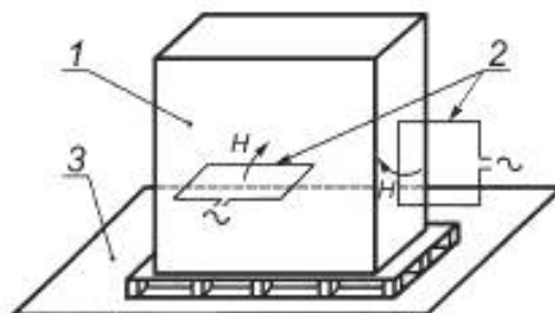
1 — ИО; 2 — индукционная катушка; 3 — эталонная пластина заземления
