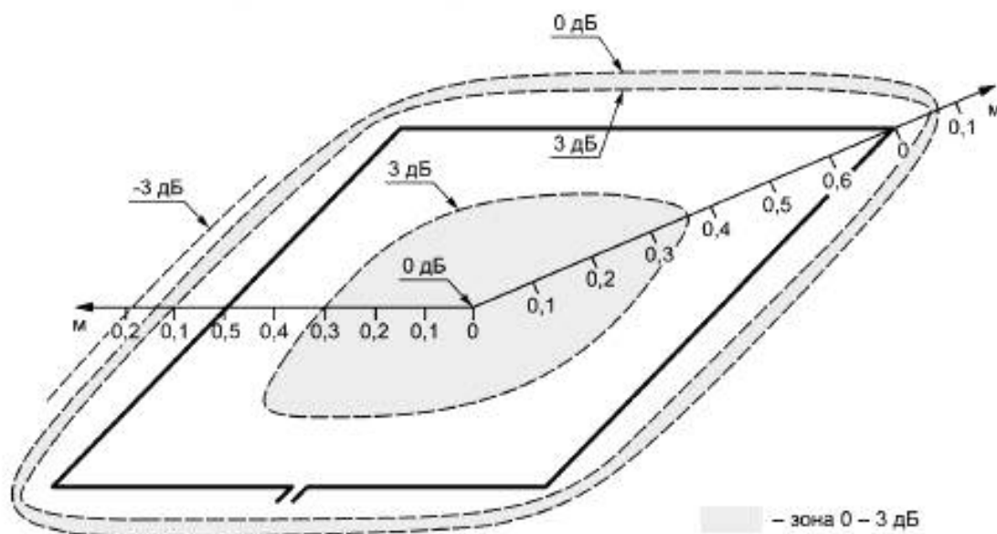
Рисунок В.2 — Зона \pm 3 дБ магнитного поля, создаваемого индукционной катушкой квадратной формы (с длиной стороны 1 м) в плоскости катушки
