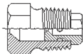
Распылительная головка в сборе
