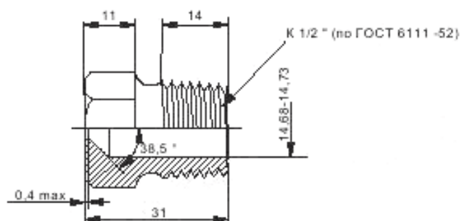
Корпус
