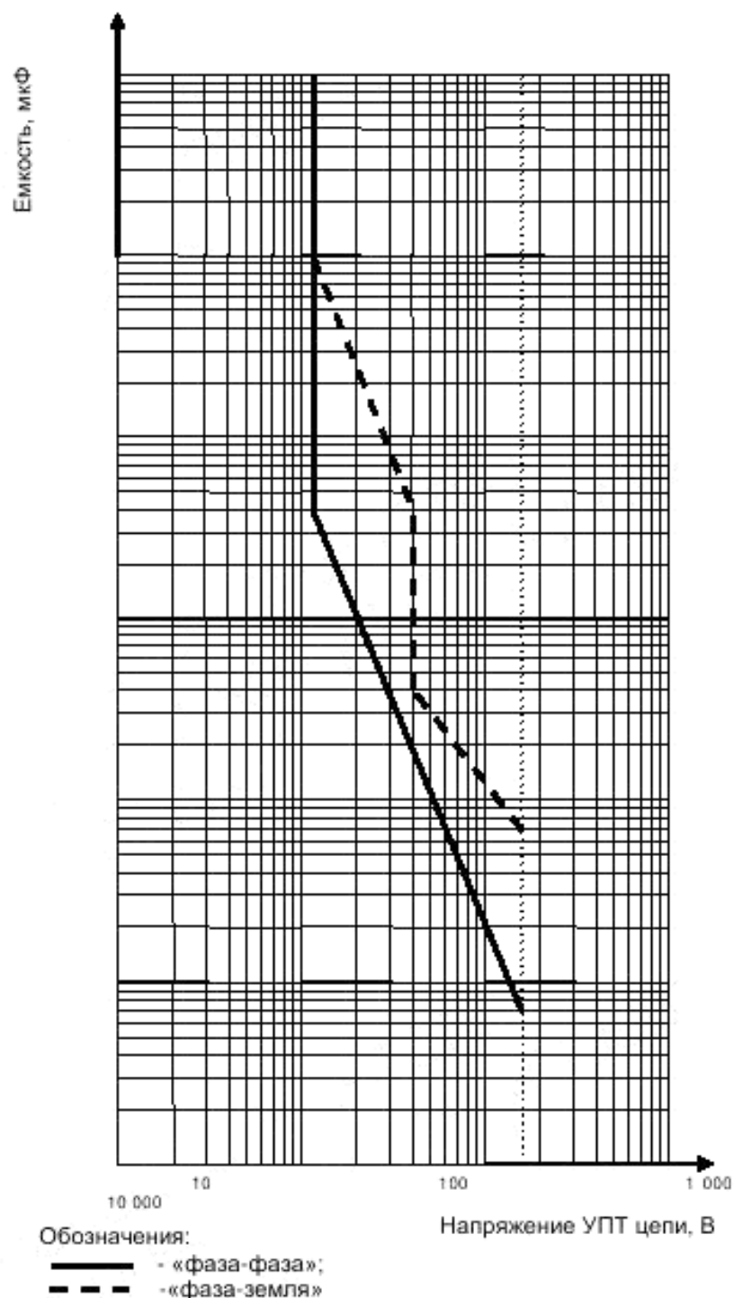
Рисунок 2 — Предельные значения для значения емкости УПТ ЦЕПИ или полной системы
