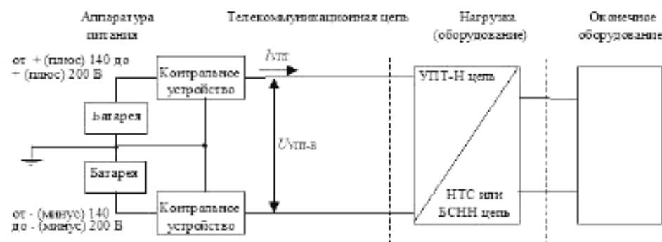
Рисунок 2 – Пример УПТ-Н системы удаленного электропитания
