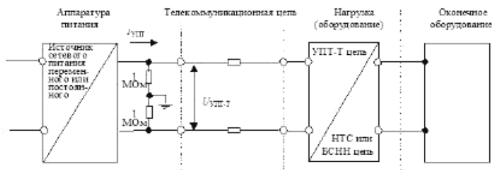
Рисунок А.1 – Пример УПТ-Т системы удаленного электропитания
