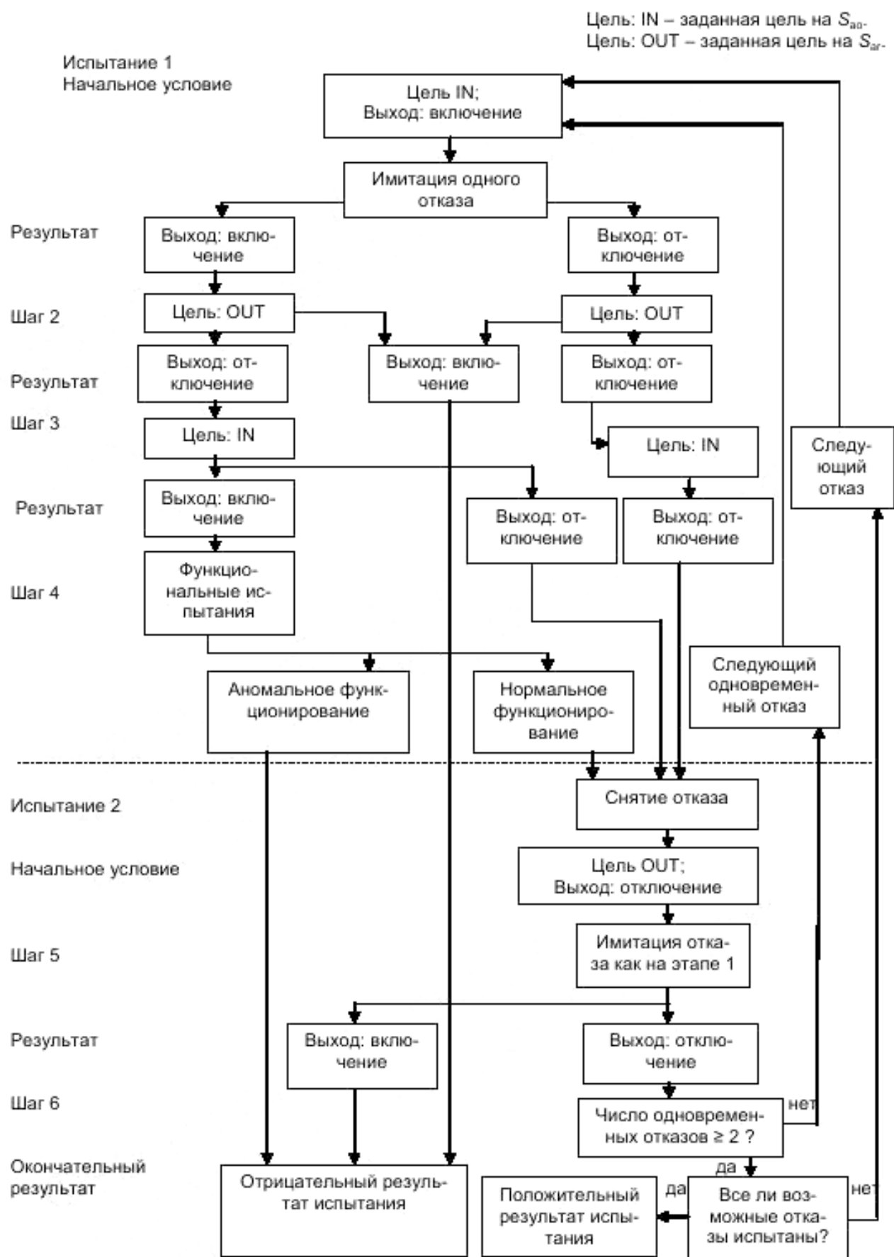
Рисунок А.3 – Последовательность испытаний для ОБД-М
