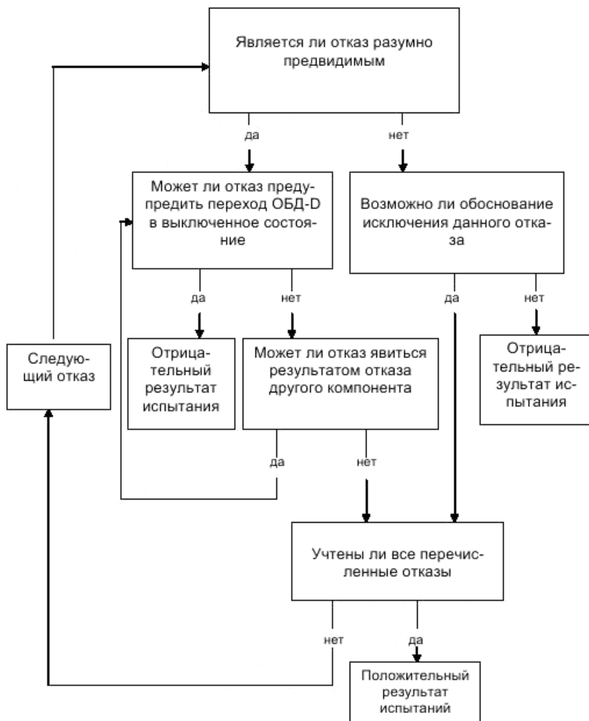
Рисунок А.1 – Оценка отказа для ОБД-D
