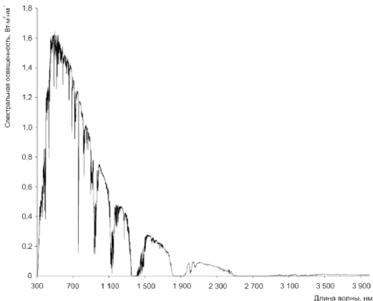
Рисунок 1 — Стандартная спектральная плотность энергетической освещенности
