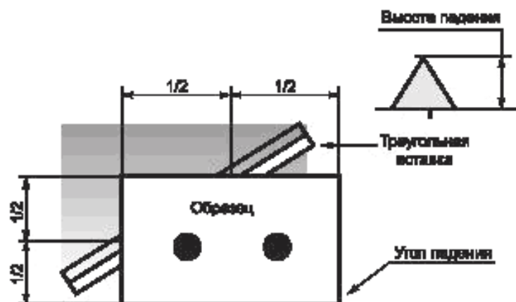
Рисунок 11 — Схема падения на угол
