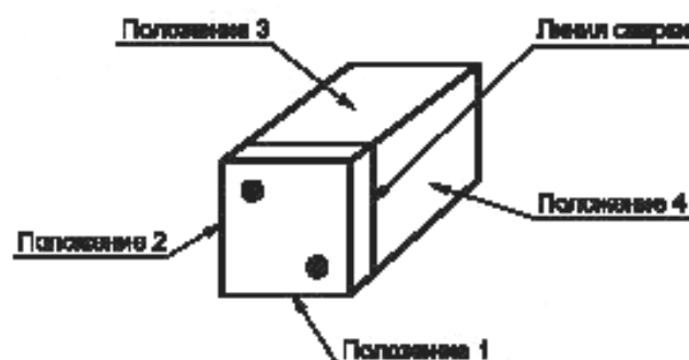
Рисунок 4 — Положение аккумулятора или моноблочной батареи при испытании
