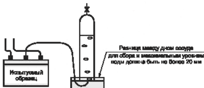
Рисунок 1 — Предполагаемое устройство для испытаний
