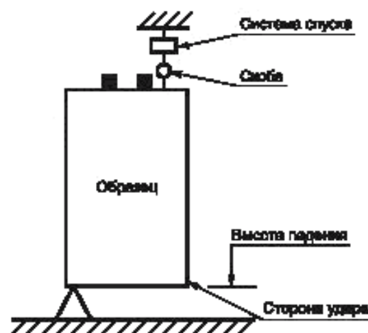
Рисунок 9 — Места на образце для удара
