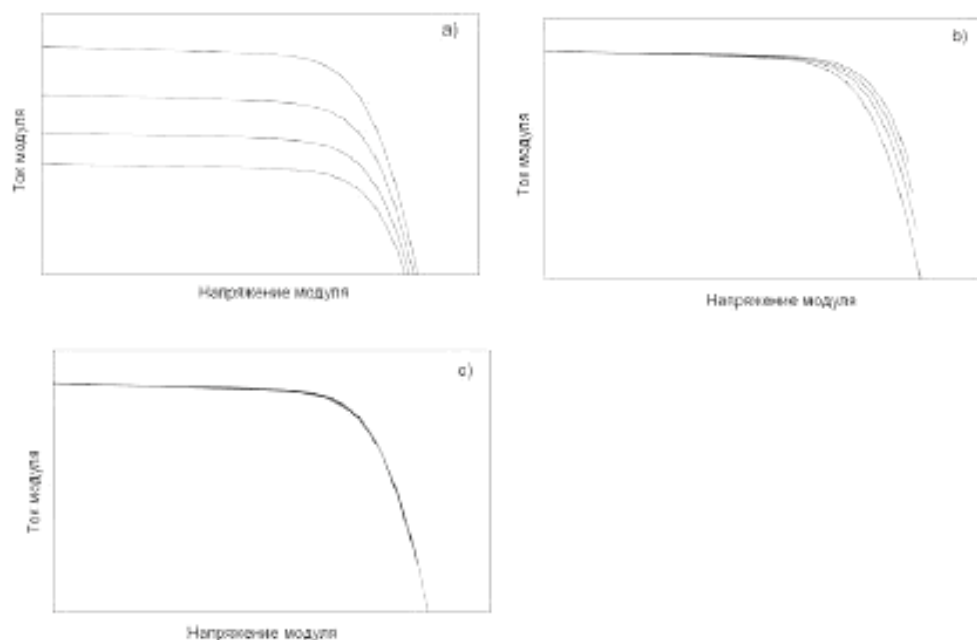
а) Графики ВАХ, измеренных при различных энергетических освещенностях и постоянной температуре; б) графики скорректированных ВАХ при R_{\text{П}} = 0 Ом; в) графики скорректированных ВАХ при найденном значении R_{\text{П}} .
