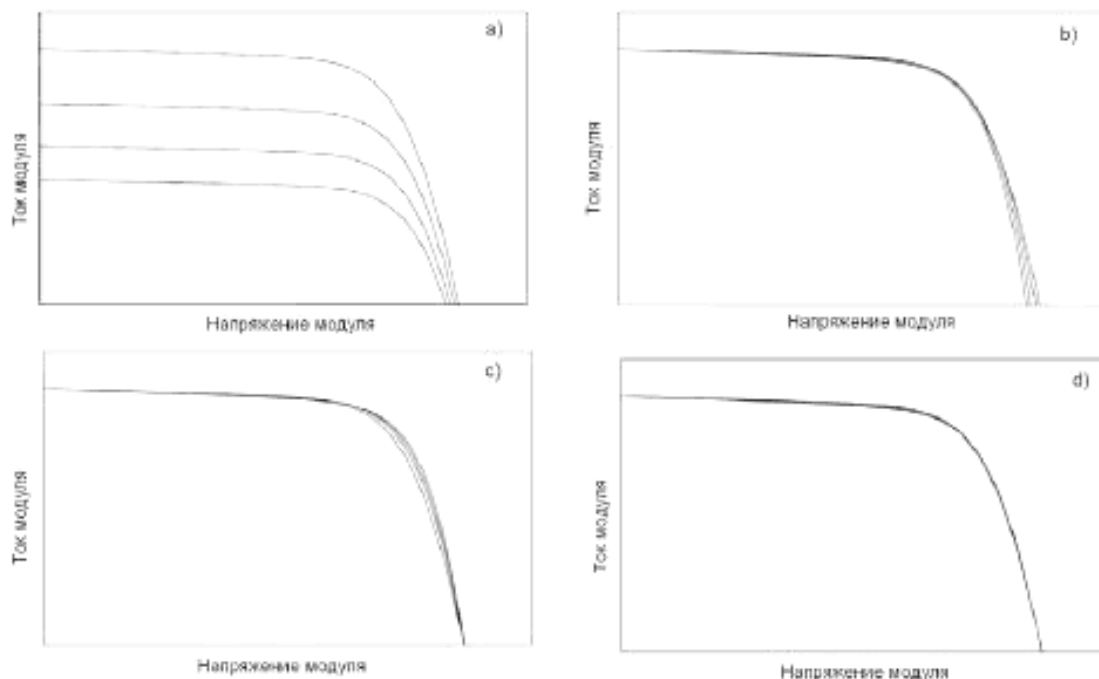
а) Графики ВАХ, измеренных при различных энергетических освещенностях и постоянной температуре; б) графики скорректированных ВАХ при a = 0 и R'_{\text{п}} = 0 Ом; в) графики скорректированных ВАХ при найденном значении a и R'_{\text{п}} = 0 Ом; г) графики скорректированных ВАХ при найденных значениях a и R'_{\text{п}} .
