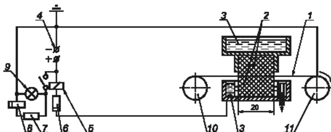
1 — провод; 2 — фетровые пластины; 3 — ванна с раствором электролита (30 г \text{Na}_2\text{SO}_4 на 1 дм воды); 4 — источник постоянного тока; 5 — реле; 6, 7 — резистор 50 кОм; 8 — счетчик; 9 — сигнальная лампа; 10 — отдающая катушка с проводом; 11 — приемная катушка
