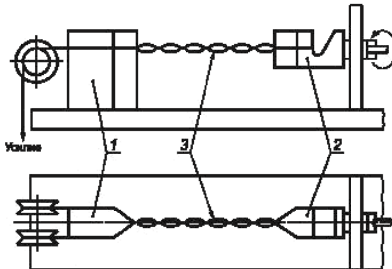
1 — неподвижная распорка; 2 — вращающийся крюк-распорка; 3 — образец
