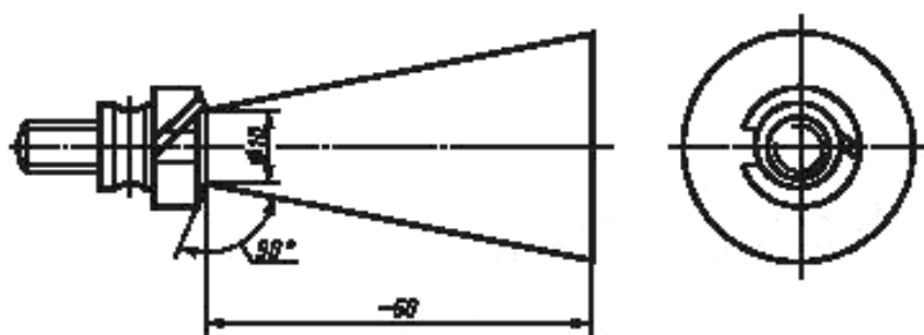
Рисунок 1 — Коническая оправка
