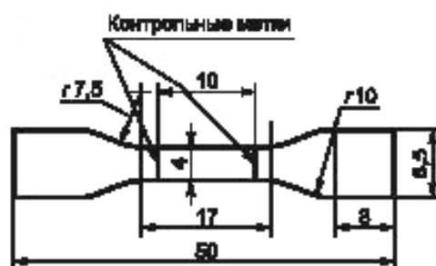
Рисунок 4 — Образец в форме двусторонней полатки небольшого размера
