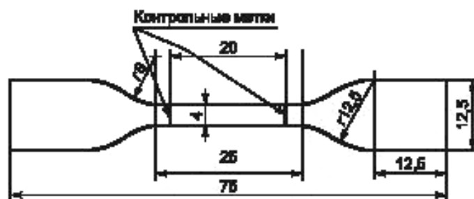
Рисунок 3 — Образец в форме двусторонней полатки
