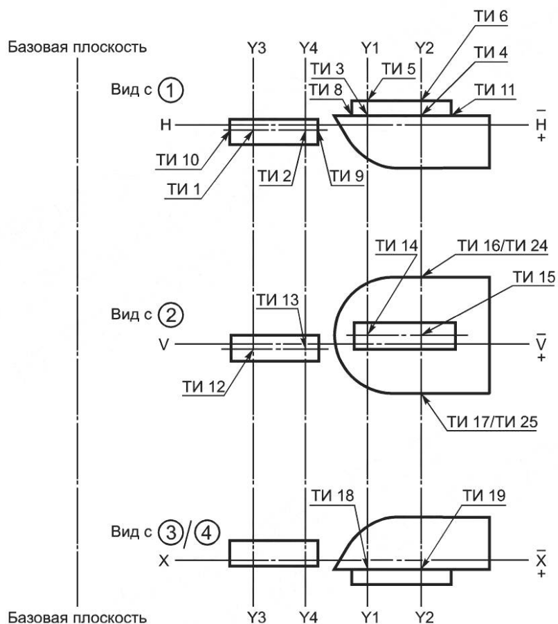
Рисунок Е.2 — Положение точек измерений
