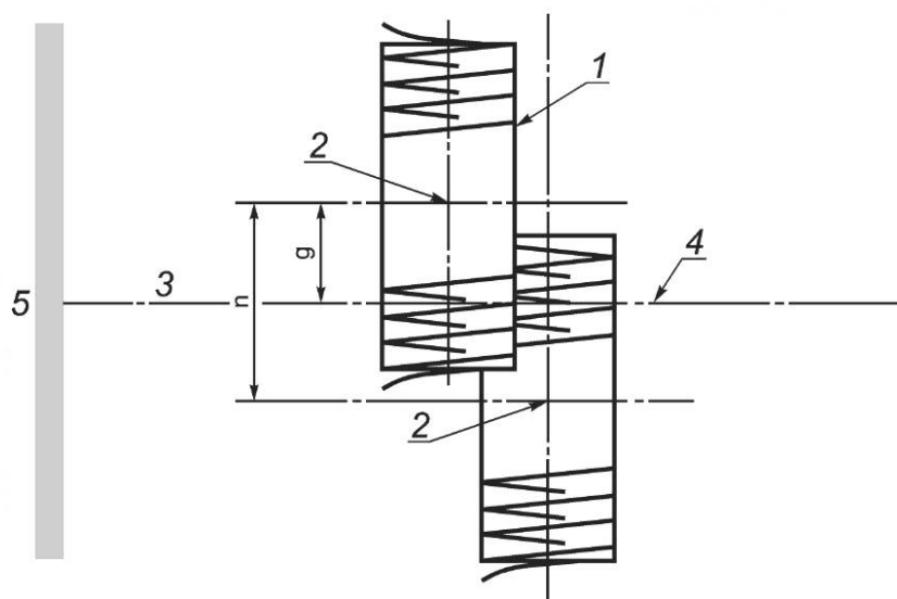
Рисунок F.1 — Вид сбоку, направление вида ③ a, b
