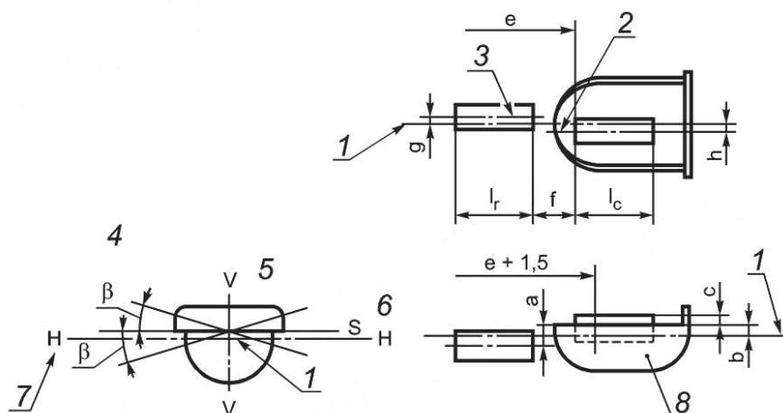
Рисунок 1 — Чертеж лампы накаливания
