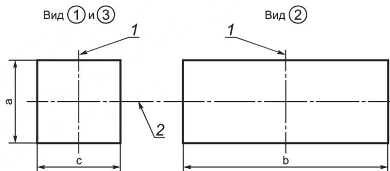
Рисунок 3 — Система проверки расположения тела накала лампы («система шаблона») [см. А.10 (приложение А)]
