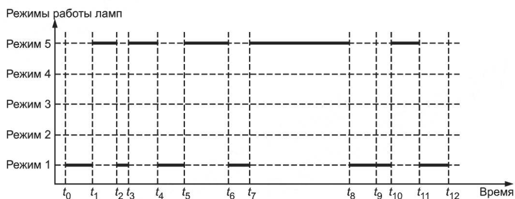
Рисунок J.7 — График переключений ламп накаливания для работы в непрерывном режиме в течение одного рабочего цикла
