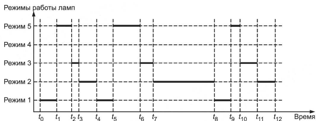
Рисунок J.8 — График переключений ламп накаливания для работы в непрерывном режиме и режимах «пульсирование» и «мигание» в течение одного рабочего цикла
