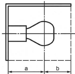
Рисунок J.1 — Схема бокса (вид сбоку)
