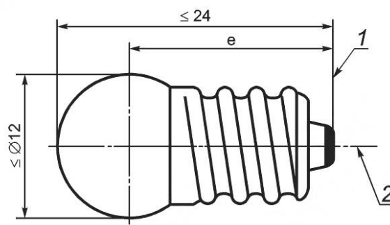
Рисунок 1 — Чертеж лампы накаливания
