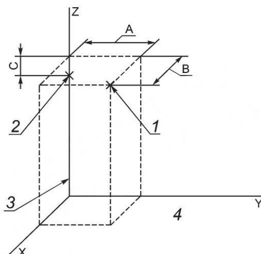
Рисунок А.3 — Схема определения боковых отклонений (А и В) и допуска на высоту светового центра (С)
