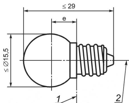
Рисунок 1 — Чертеж лампы накаливания
