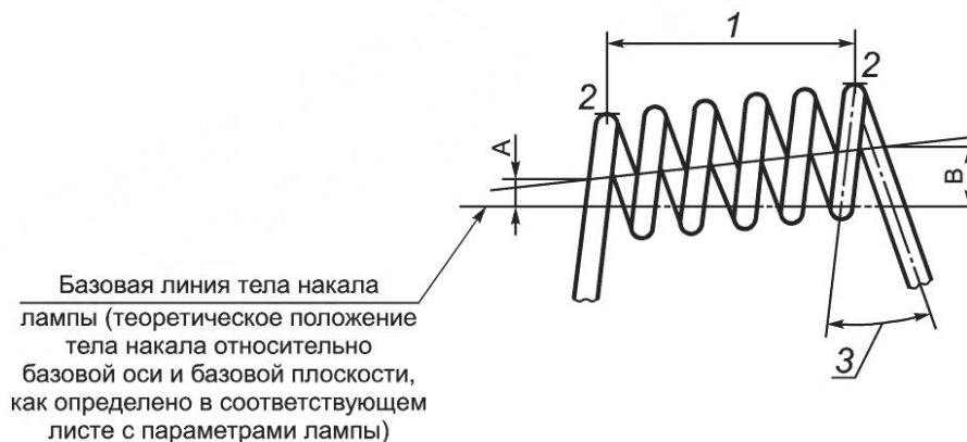
Рисунок А.1 — Схема определения вершин, длины и смещений тела накала лампы (А и В)
