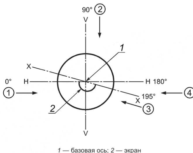
Рисунок Е.1 — Направления видов, вид лампы сверху
