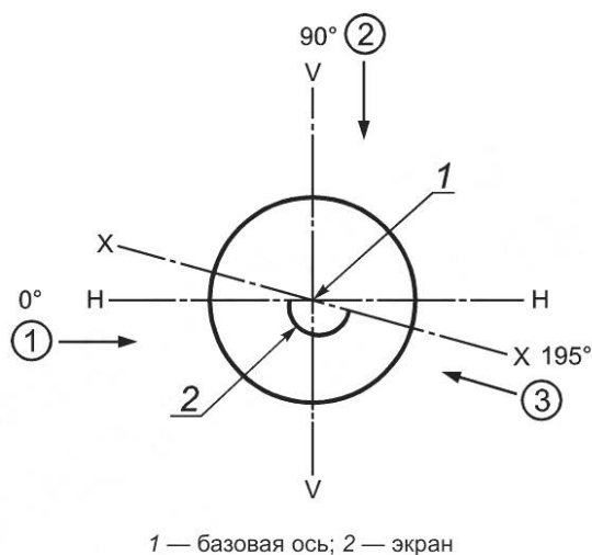
Рисунок D.1 — Направления видов, вид лампы сверху
