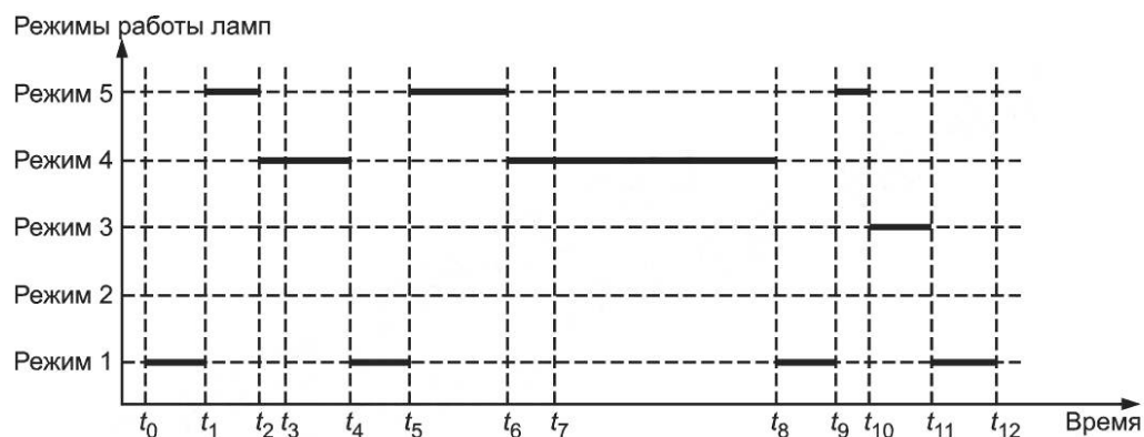
Рисунок J.6 — График переключений ламп накаливания для работы в непрерывном режиме и режиме «прерывание» в течение одного рабочего цикла
