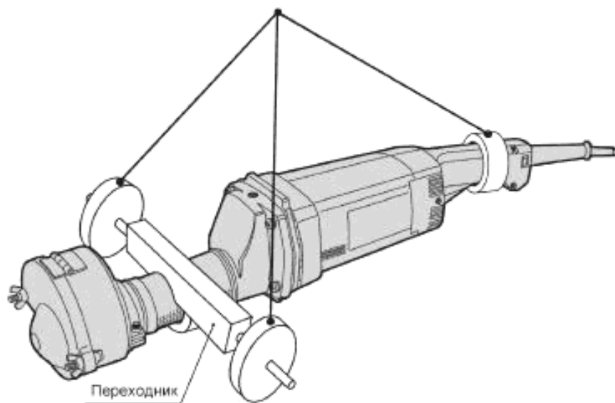
Рисунок 109 — Испытание кожуха на прочность: прямая шлифовальная машина с дополнительными массами
