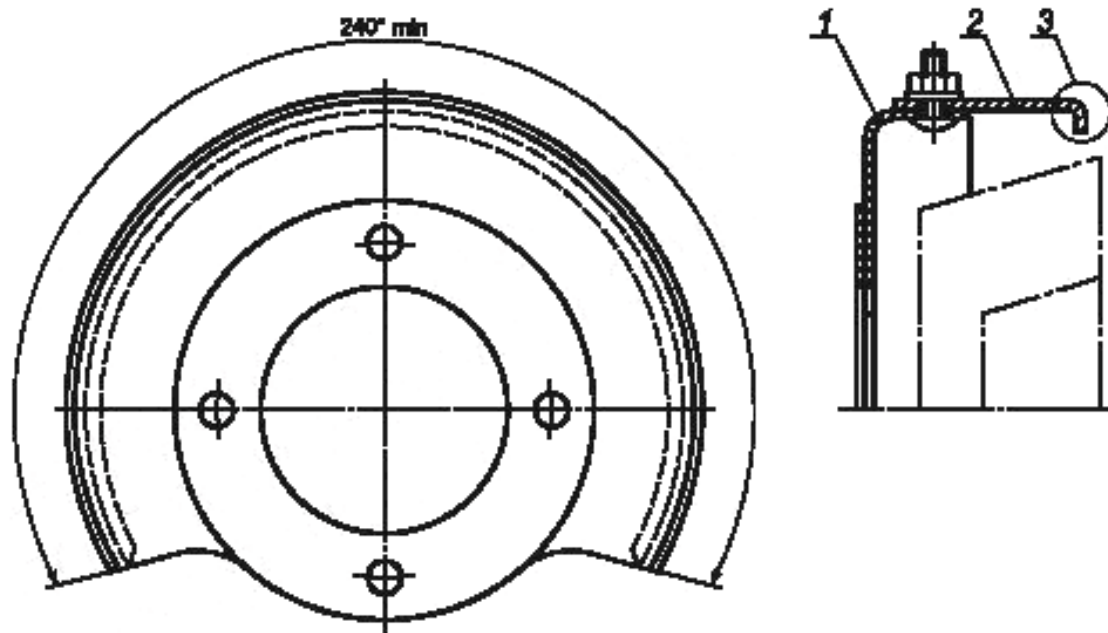
Рисунок 103 — Регулируемый кожух для чашечного круга типов 6 и 11
