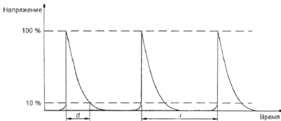
Рисунок 101 – Генерация импульсов искрового зажигания
