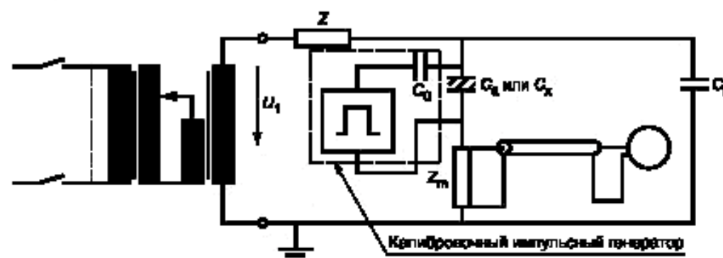
U_1 — испытательное напряжение; Z — фильтр; C_0 — емкостное сопротивление калибровочного генератора импульсов; C_d или C_k — испытуемый образец (обычно он может быть емкостным сопротивлением); C_k — накопительный конденсатор; Z_m — измерительный импеданс
