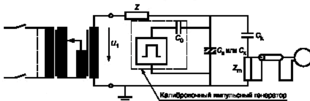
U_1 — испытательное напряжение; Z — фильтр; C_0 — емкостное сопротивление калибровочного генератора импульсов; C_d или C_k — испытуемый образец (обычно он может быть емкостным сопротивлением); C_k — накопительный конденсатор; Z_m — измерительный импеданс
