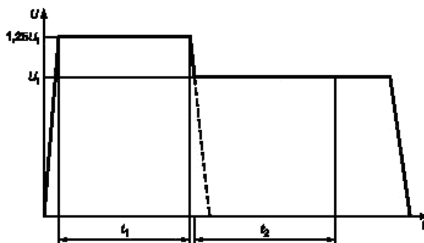
Рисунок 3 – Испытательное напряжение
