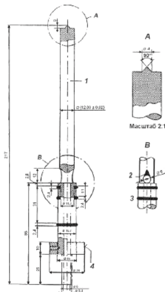
1 – внутренний электрод; 2 – отметка заполнения; 3 – уплотнительные кольца внешним диаметром 16,1 мм и внутренним диаметром 11,3 мм; 4 – rifленая поверхность
