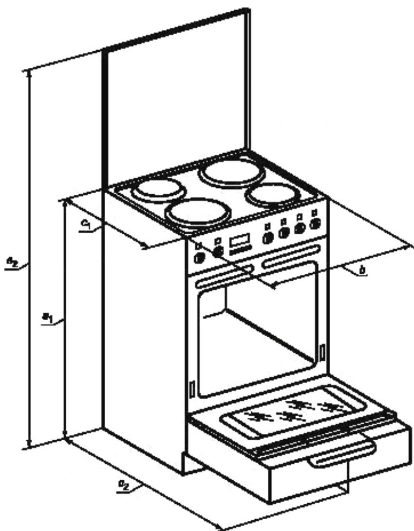
Рисунок 1 — Размеры приборов
