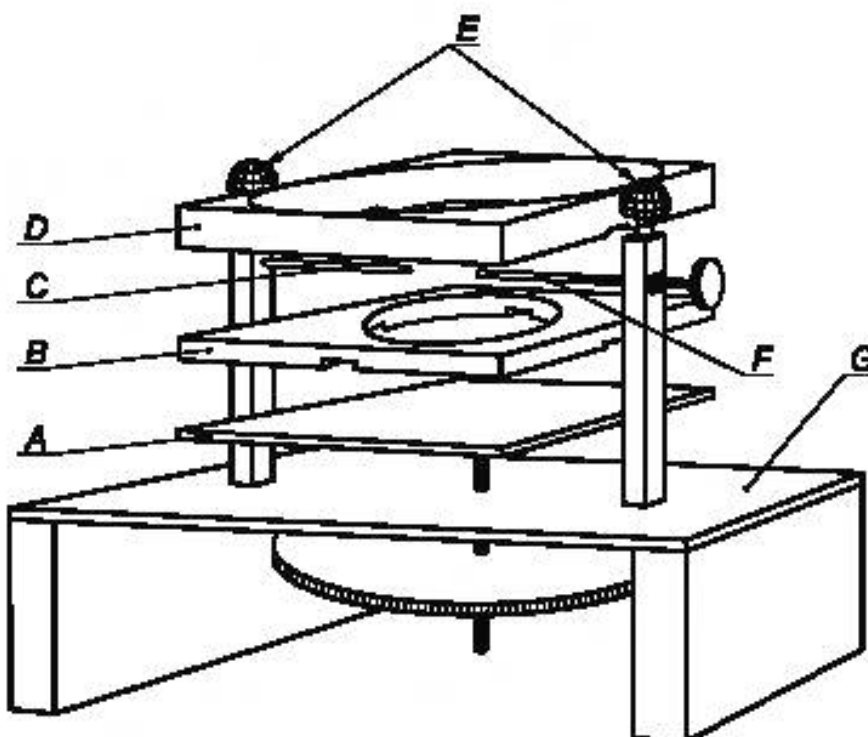
А — регулируемая платформа; В — нижняя часть щита (см. деталь А на рисунке 104); С — неподвижный электрод; D — верхняя часть щита (см. деталь В на рисунке 104); E — зажимы; F — подвижный электрод; G — основная плита
