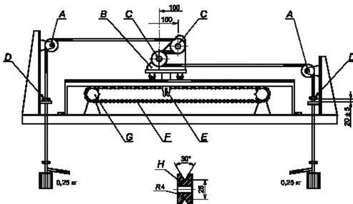
А — шкив диаметром > 50 мм; В — тележка; С — шкив с желобком; D — удерживающий зажим; E — сцепляющий штырь; F — цепь с шагом 12,7 мм; G — цепное колесо с 20 зубцами диаметром начальной окружности 88,9 мм; H — подробно о шкиве С
