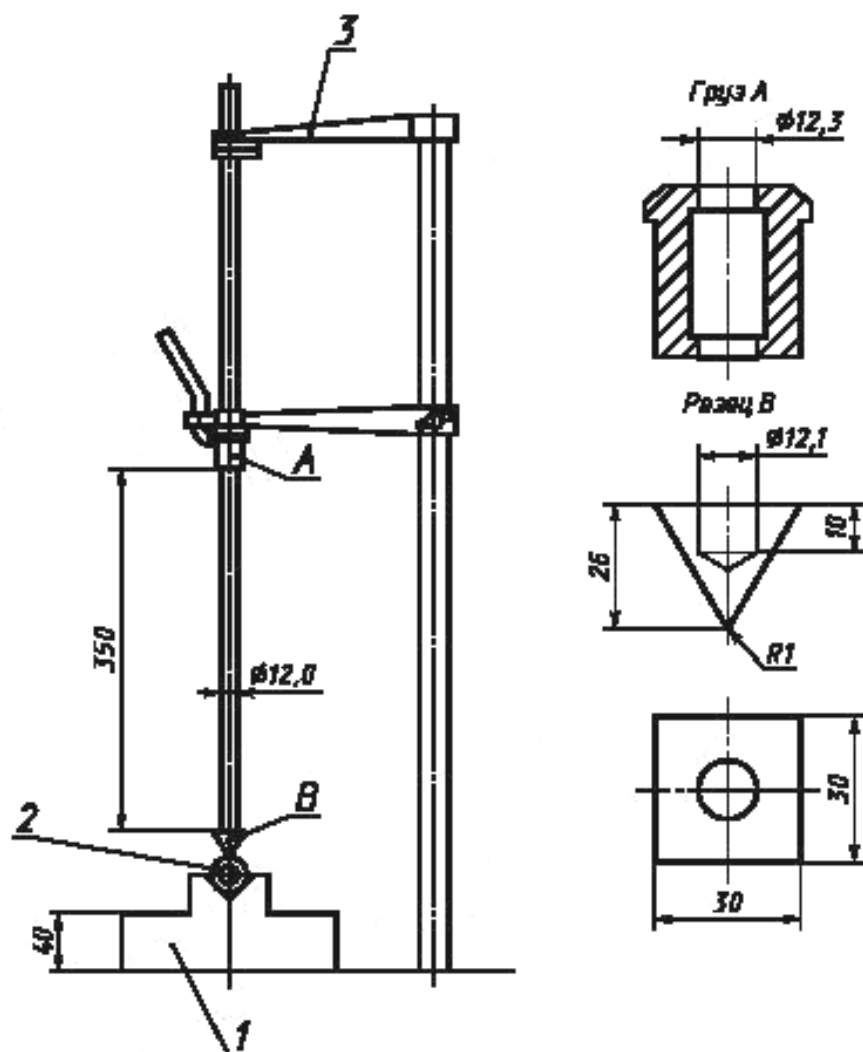
1 — основание массой 10 кг; 2 — образец; 3 — фиксирующий кронштейн
