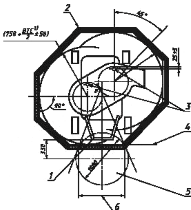
Рисунок ВВ.3 — Многошпиндельная косилка. Испытательное ограждение
