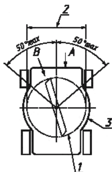
1 — траектория лезвия; 2 — ширина лезвия; 3 — ограждение лезвия
