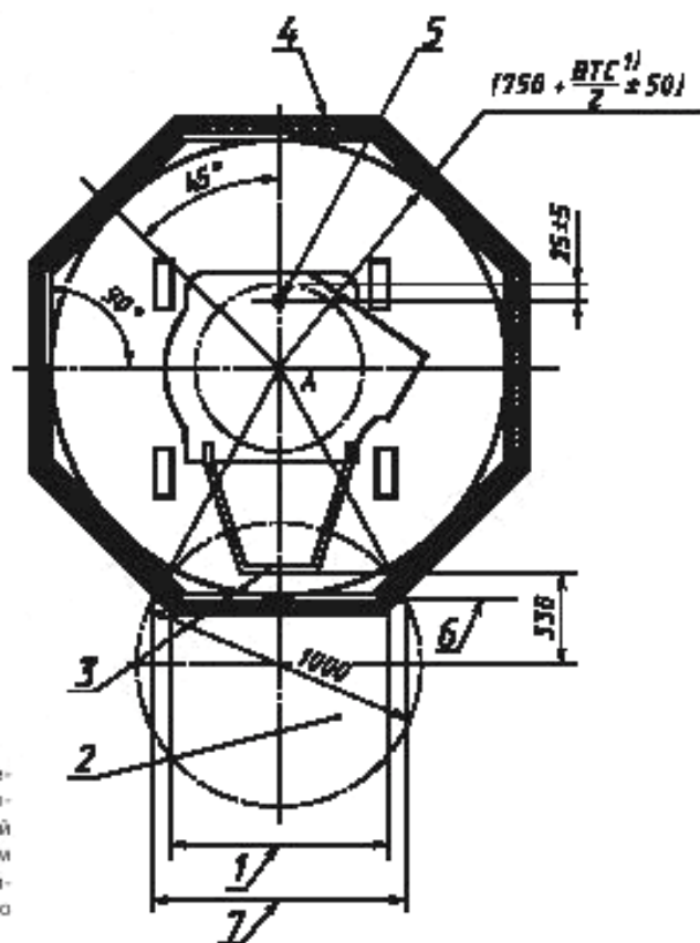
Рисунок ВВ.2 — Одношпindleльная косилка. Испытательное ограждение
