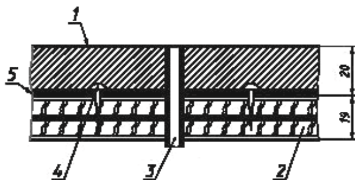
1 — коврик из кокоса; 2 — основание из фанеры; 3 — труба для выброса; 4 — гвоздь; 5 — поливинилхлоридное основание
