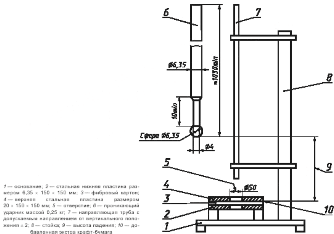
Рисунок ВВ.5 — Испытательный стенд для проверки проникания через фибровый картон
