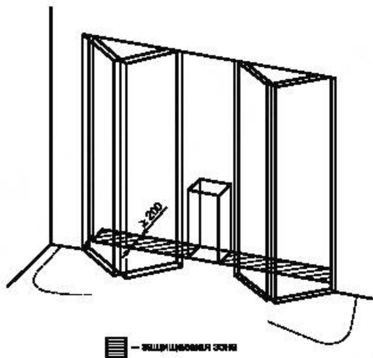
Рисунок EE.5 — Складывающийся дверной блок
