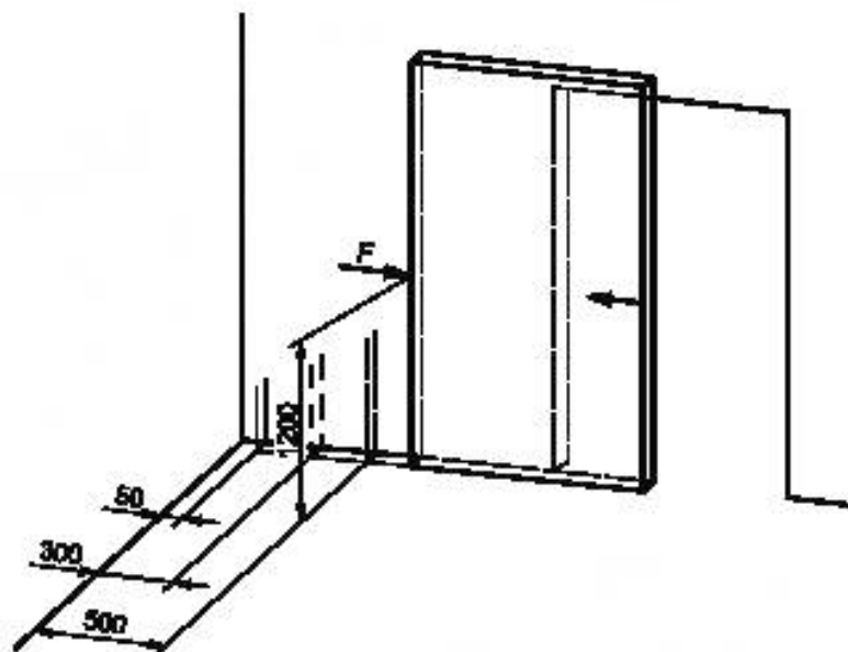
Рисунок II.1 — Одностворчатый раздвижной дверной блок
