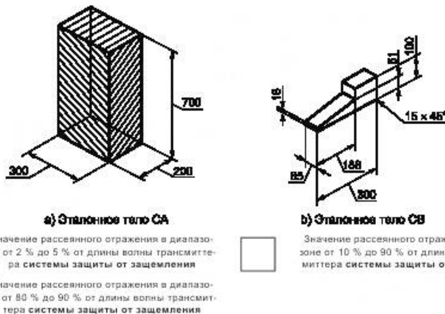
Рисунок FF.1 — Эталонные тела
