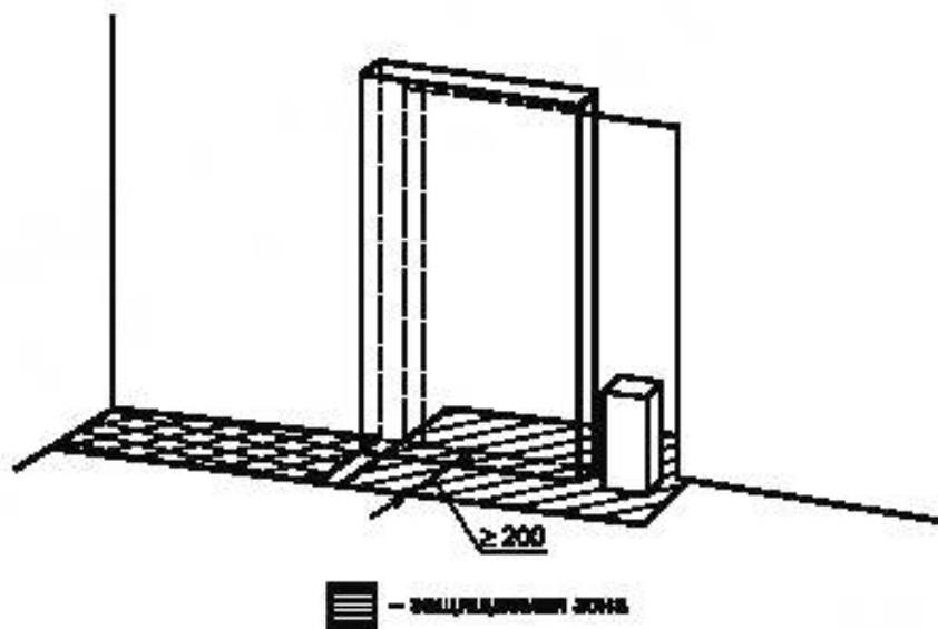
Рисунок ЕЕ.1 — Одностворчатый раздвижной дверной блок
