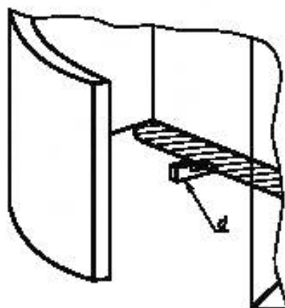
a) Положения эталонного тела для испытания 1 и испытания 2
