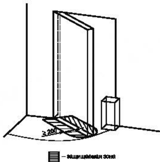
Рисунок ЕЕ.3 — Одностворчатый распашной дверной блок
