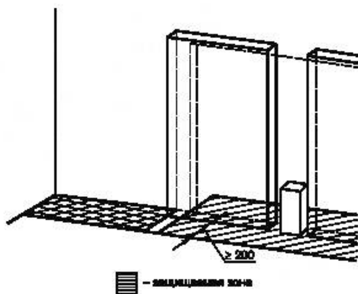
Рисунок ЕЕ.2 — Двустворчатый раздвижной дверной блок
