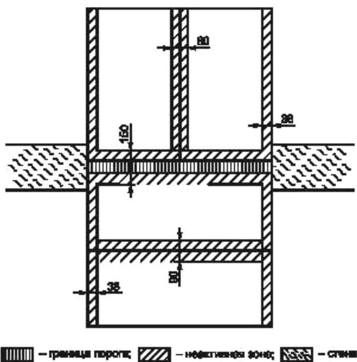
Рисунок 102 — Неактивные зоны на полу чувствительных к давлению кнопок
