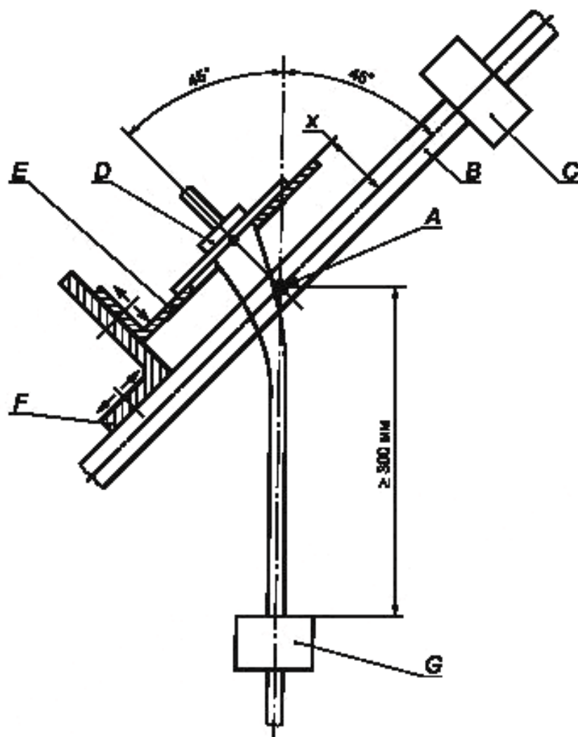
Рисунок 8 – Устройство для испытания на изгиб
