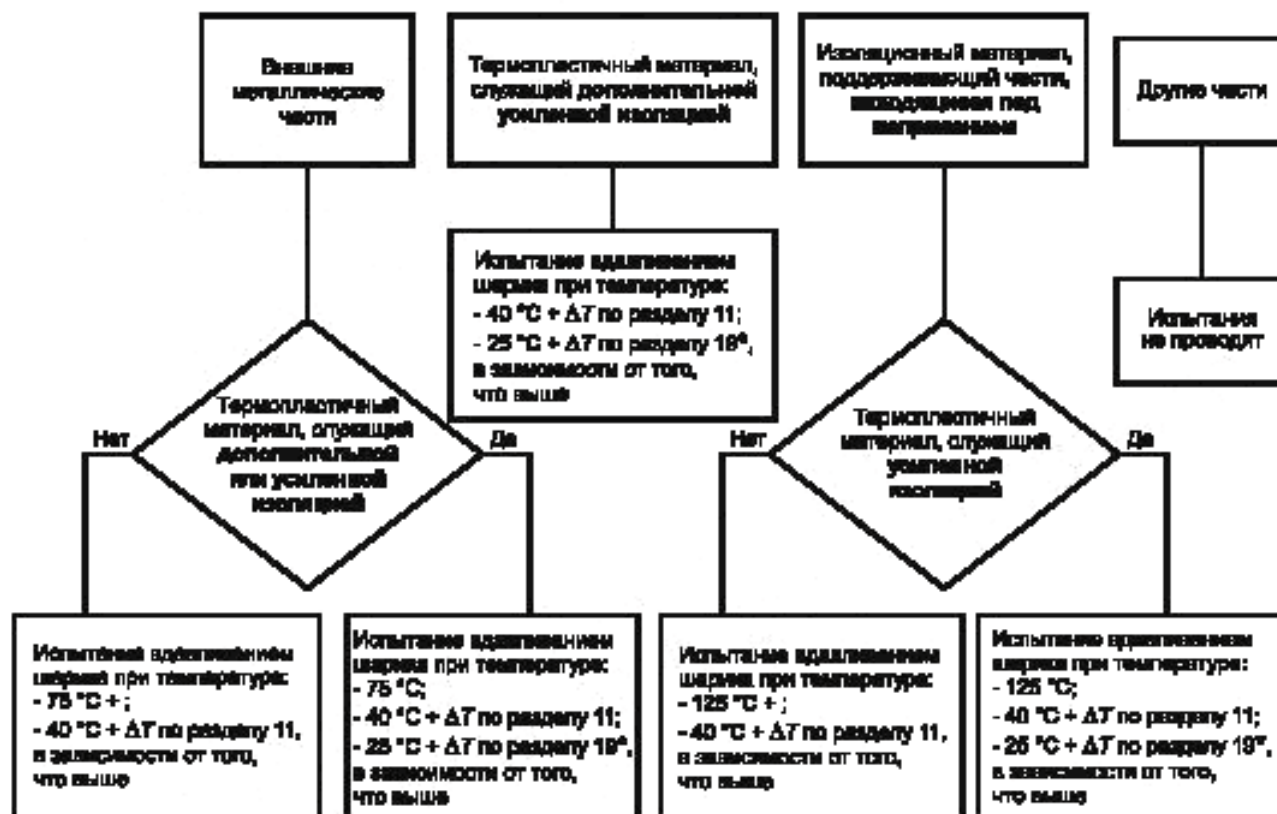
Рисунок О.1 – Испытания на теплостойкость
