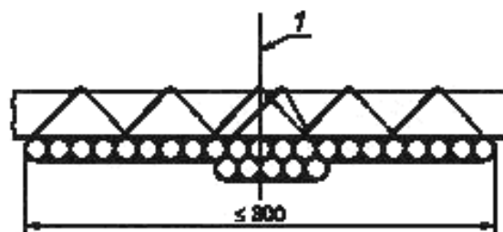
1 — центральная линия лестницы
