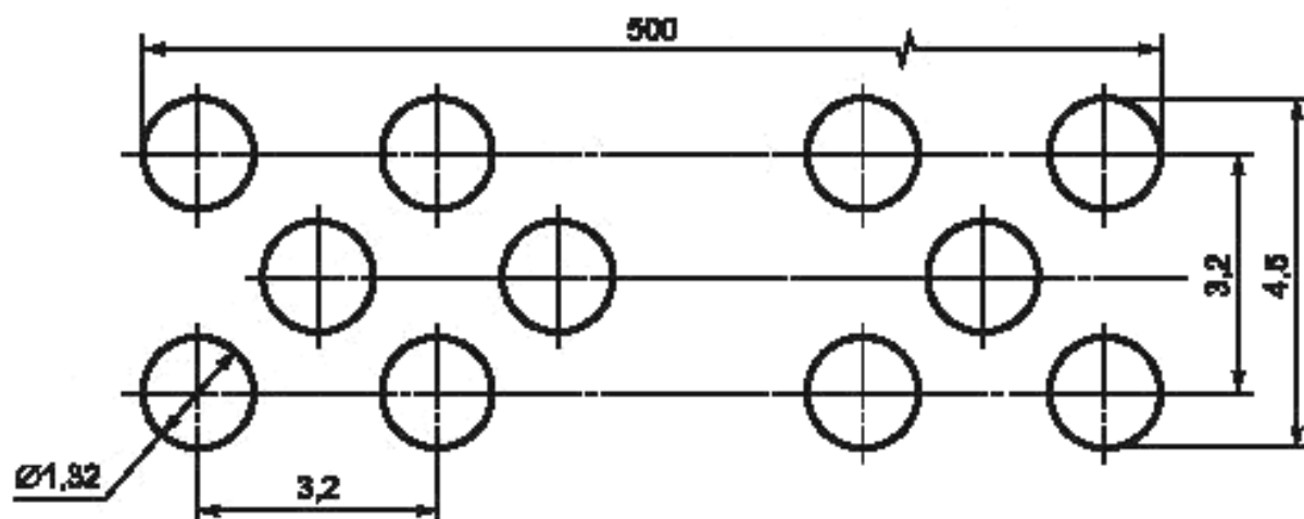
Рисунок 2 — Фронтальная поверхность рабочей части горелки
