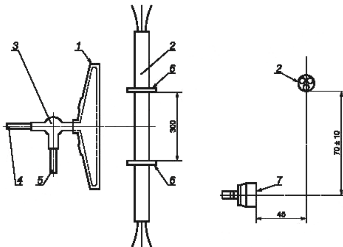
1 — горелка; 2 — образец кабеля; 3 — смеситель Вентури; 4 — подача воздуха; 5 — подача пропана; 6 — поддерживающие кольца; 7 — фронтальная поверхность рабочей части горелки
