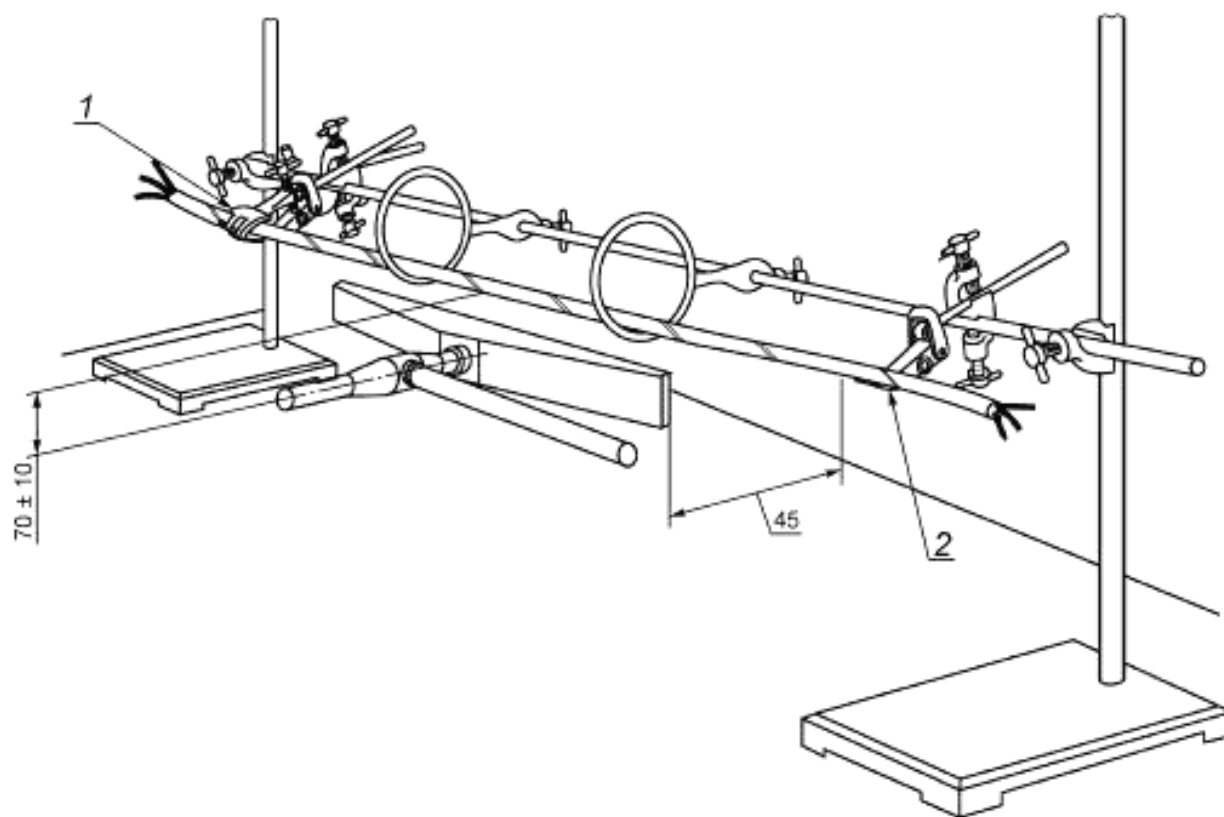
1 — зажим; 2 — опора
