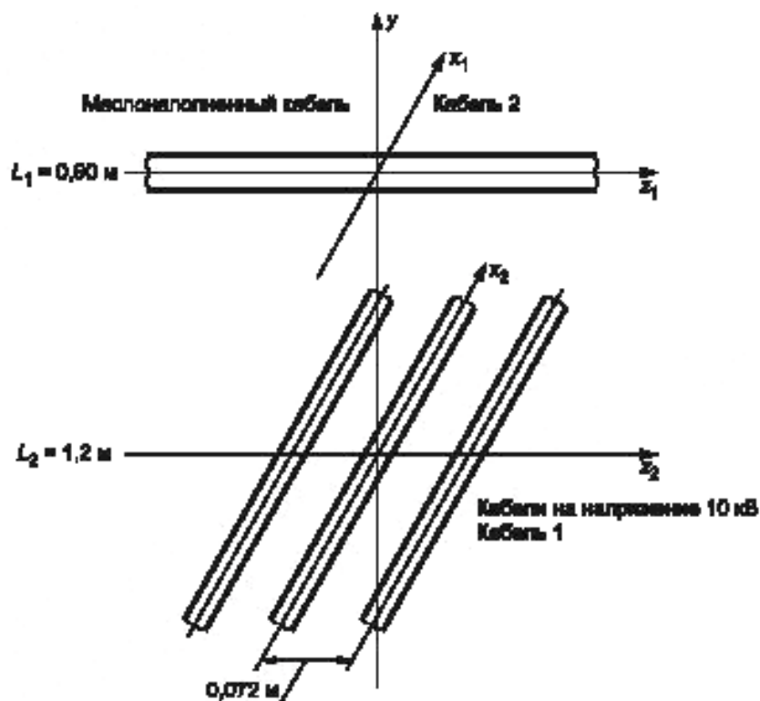
Рисунок А.1 — Расположение кабелей
