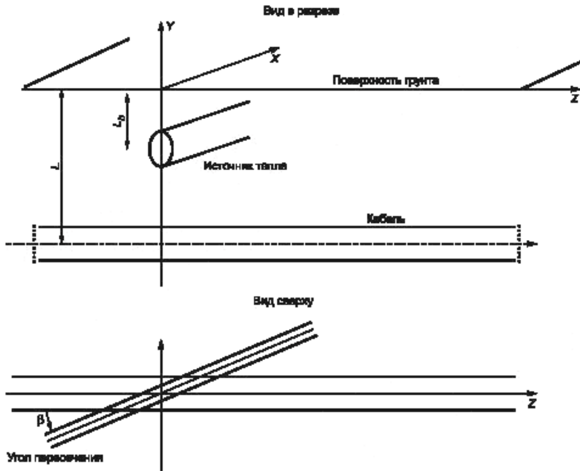
Рисунок 1 — Пример расположения источника тепла, пересекающего рассматриваемый кабель
