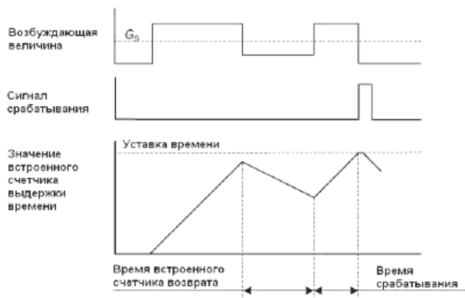
Рисунок В.1 — Определение зависимости времени возврата
