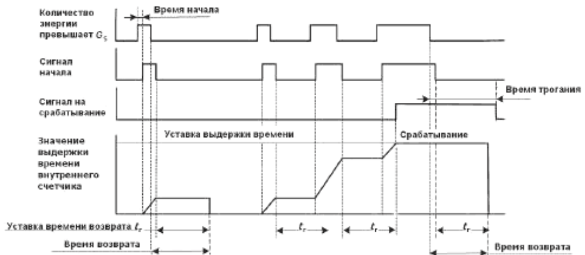
Рисунок 5 — Характеристика, поясняющая время возврата реле
