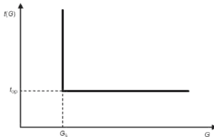
Рисунок 2 — Независимая характеристика времени реле сверхтока
