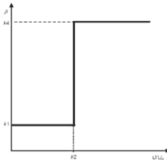
Рисунок 10 — Характеристика управляющего напряжения
