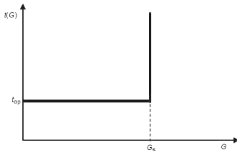
Рисунок 3 — Независимая характеристика времени реле минимального тока
