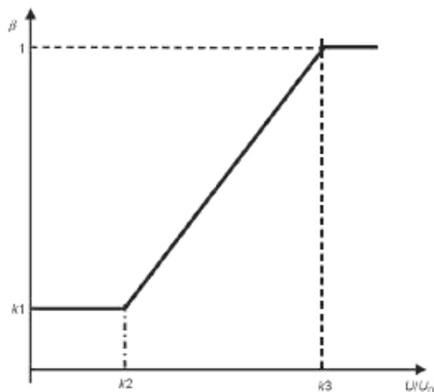
Рисунок 9 — Характеристика ограничения напряжения
