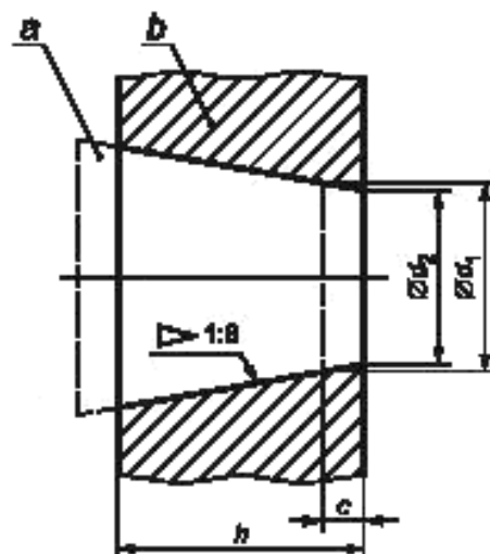
а — конусный кабельный наконечник; б — конусное гнездо
