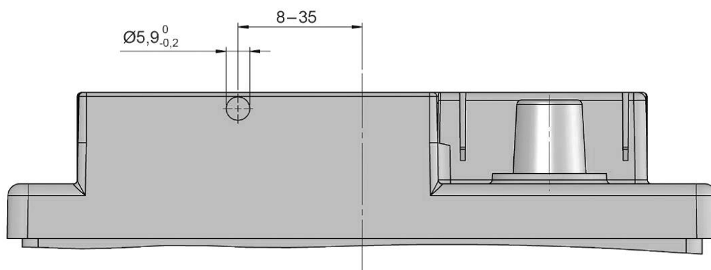
Рисунок 10 — Размеры отверстий системы дегазации
