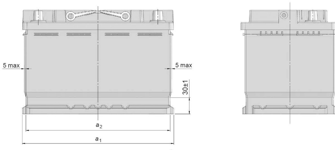
Рисунок 17 — Размеры допустимого утолщения боковых стенок корпуса на коротких сторонах батареи
