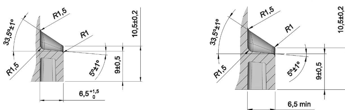
а) Размеры деталей бортика на длинной стороне корпуса батареи (вертикальный разрез М-М)
