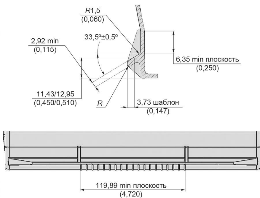
Рисунок 32 — Форма и размеры углублений на корпусе, образующих бортик на короткой стороне корпуса батареи
