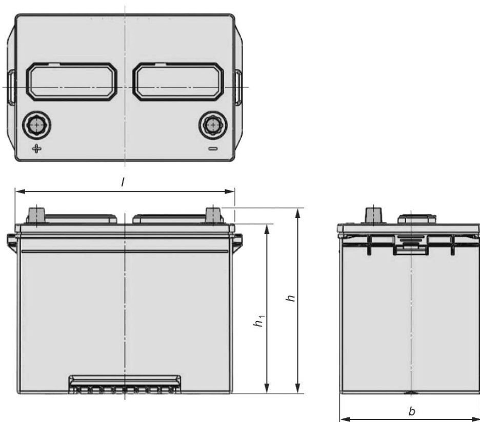
Рисунок 36 — Основные размеры батарей типоразмеров 24, 25, 26, 27, 34, 51, 86
