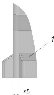
a) Размеры детали K
