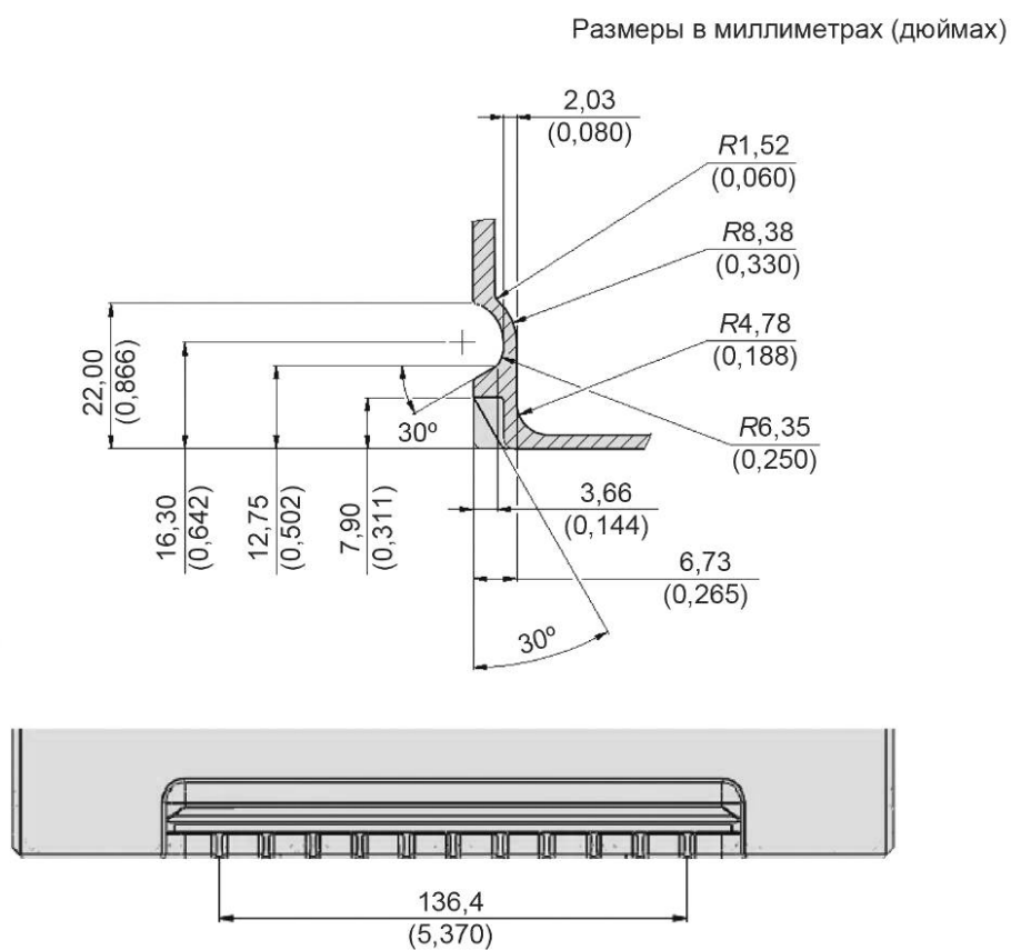
Рисунок 33 — Форма и размеры углублений на корпусе, образующих бортик на короткой стороне корпуса батареи
