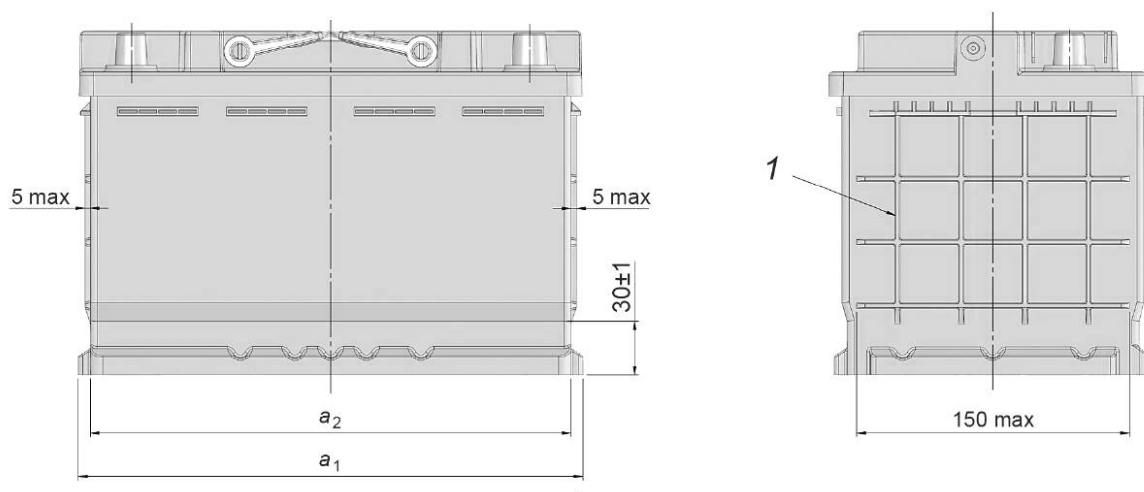
Рисунок 18 — Допустимая высота ребер жесткости на коротких сторонах батареи
