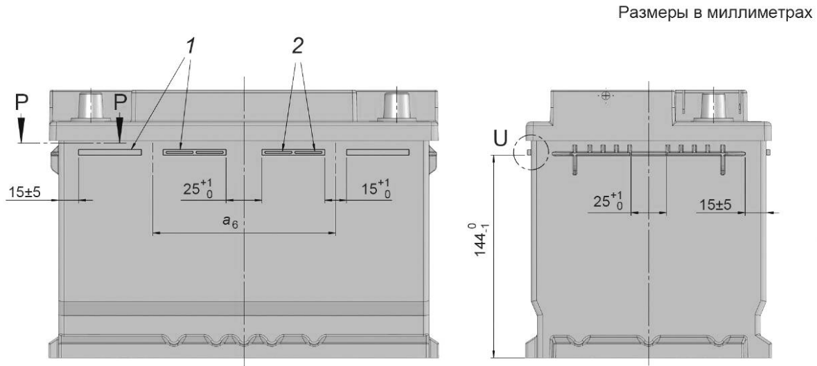
Рисунок 13 — Месторасположение выступов для ЗРО с учетом размеров, указанных в таблице 1 (допускаются оба варианта исполнения выступов) 2)
