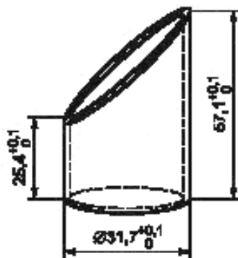
Рисунок 7 — «Глотабельный» калибр
