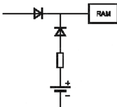
Рисунок 6 — Схема соединений для обеспечения защиты от заряда
