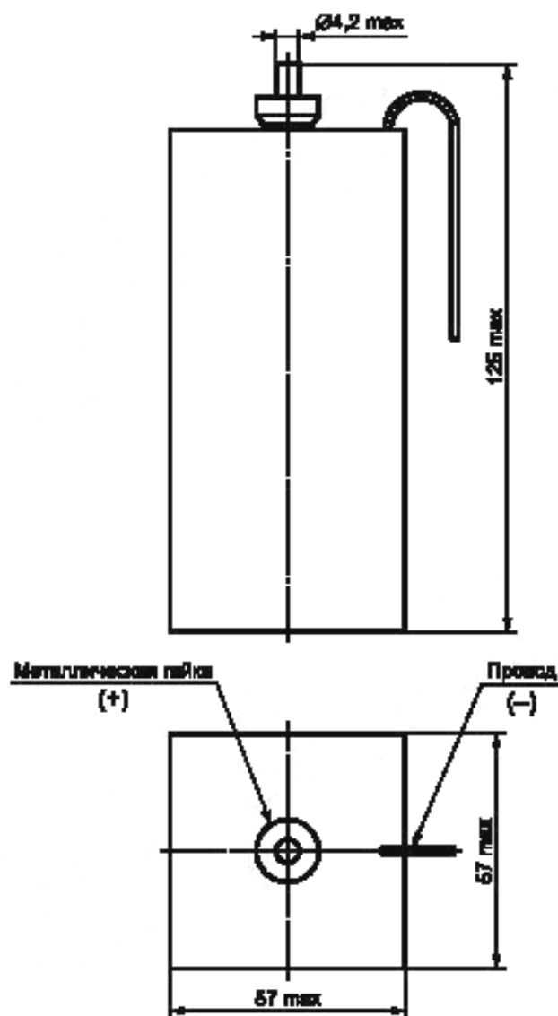
Рисунок 9 — Размеры батареи S4
