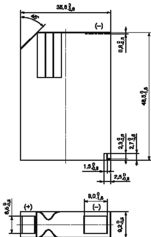
Рисунок 11 — Размеры батарей 4LR61
