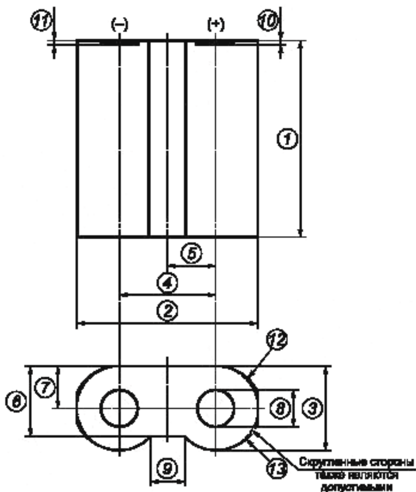
Рисунок 12 — Размеры батарей CR-P2, BR-P2
