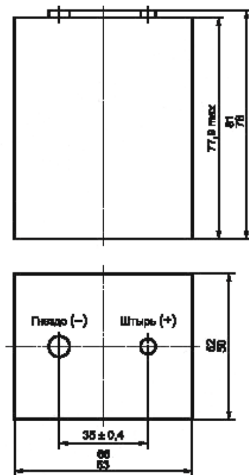
Рисунок 21 — Размеры батареи 6F100
