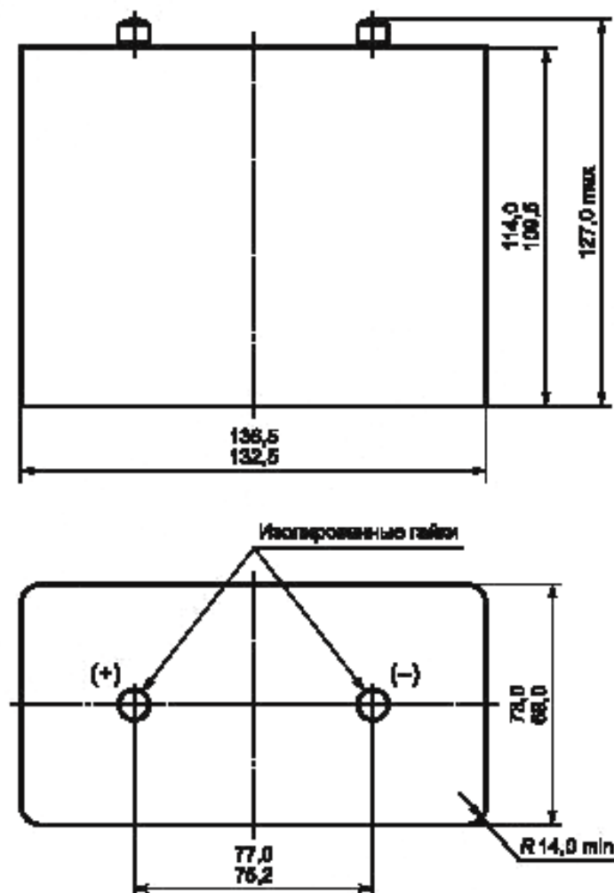
Рисунок 17 — Размеры батарей 4R25-2, 4LR25-2
