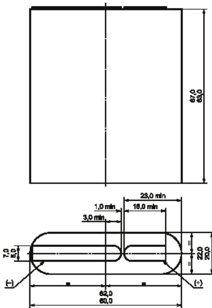
Рисунок 10 — Размеры батарей 3R12C, 3R12P, 3R12S, 3LR12
