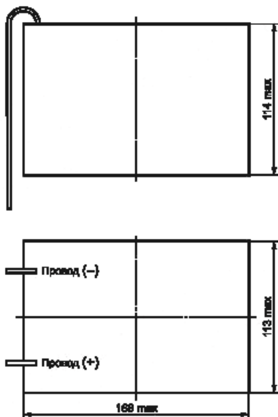
Рисунок 18 — Размеры батареи 6AS4
