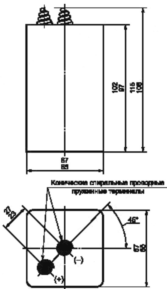
Рисунок 15 — Размеры батарей 4R25X, 4LR25X
