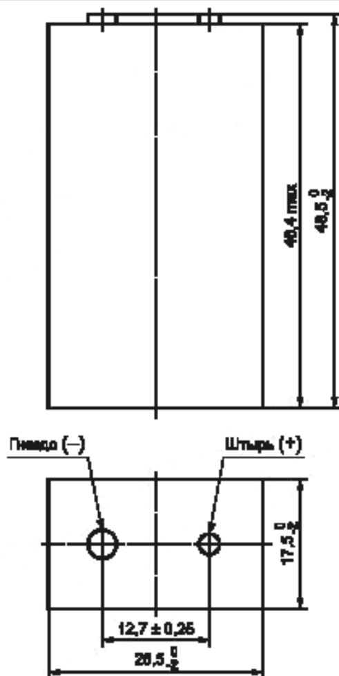
Рисунок 20 — Размеры батарей 6F22, 6LR61
