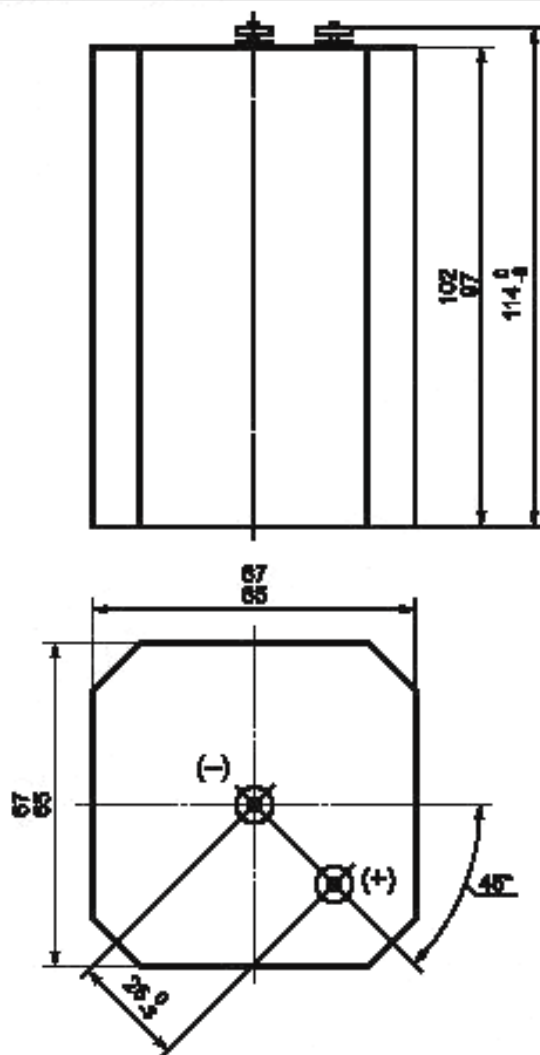
Рисунок 16 — Размеры батареи 4R25Y
