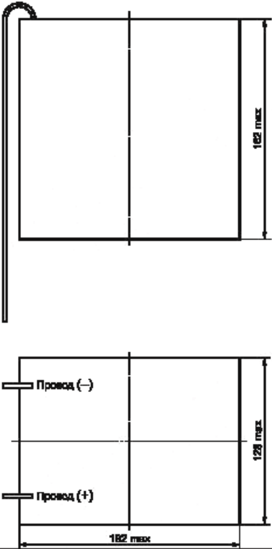
Рисунок 19 — Размеры батареи 6AS6
