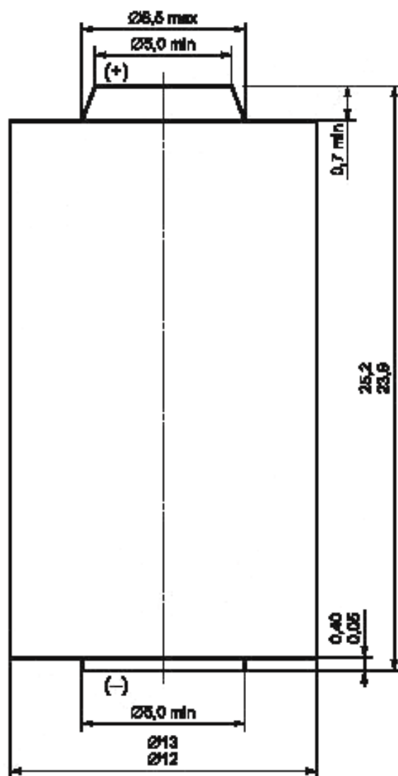
Рисунок 7 — Размеры батарей 4LR44, 2CR13252, 4SR44
