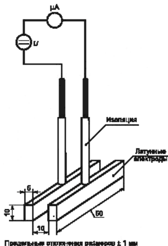
Рисунок 1 — Испытательная установка для определения диэлектрических свойств заполнителя
