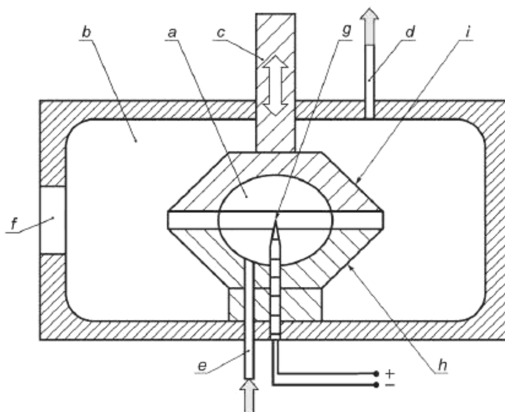
a — внутренняя сферическая камера; b — внешняя цилиндрическая оболочка; c — регулируемая часть (микрометрический винт); d — выходное отверстие; e — входное отверстие; f — смотровое окно; g — искровой электрод; h — нижняя стационарная поверхность зазора; i — верхняя регулируемая поверхность зазора
