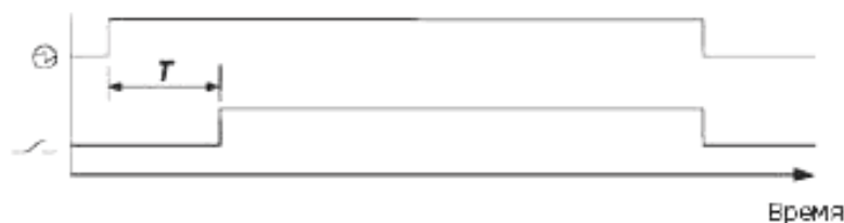
⊙ – источник электропитания; T – установленное время; / – главный контакт Рисунок 1 – Реле с задержкой по включению электропитания
