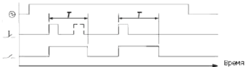
⊕ – источник электропитания; \downarrow – сигнал управления; T – установленное время; — — рабочий контакт
