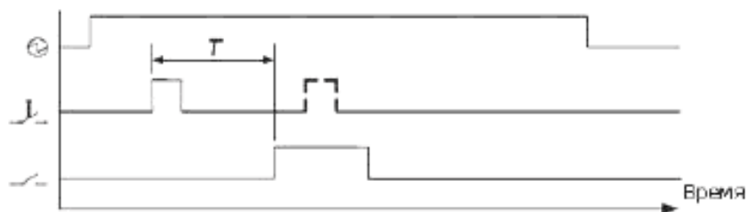
⊕ – источник электропитания; I – сигнал управления; T – установленное время; ⏏ – рабочий контакт Рисунок 9 – Импульсное реле с задержкой по управляющему сигналу
