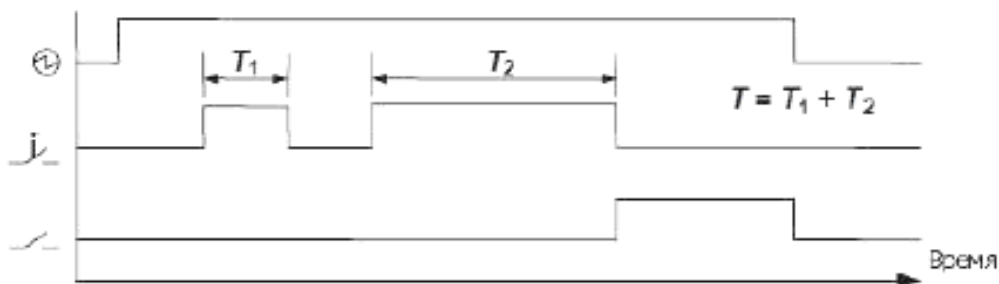
Рисунок 7 – Реле время суммирования
