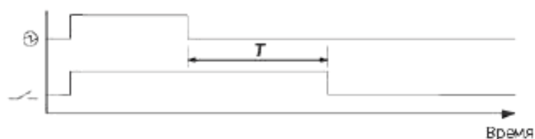
Ⓢ – источник электропитания; T – установленное время; J – главный контакт Рисунок 2 – Реле с задержкой по выключению электропитания
