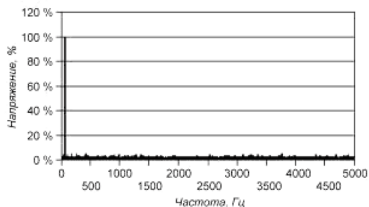
Спектр частот напряжения на выходе преобразователя — инвертора напряжения типа В, f_1 = 50 Гц, f_{ср.} = 4,5 кГц
