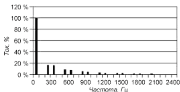
Спектр частот тока на выходе 6-пульсного преобразователя — инвертора тока, f_1 = 50 Гц
