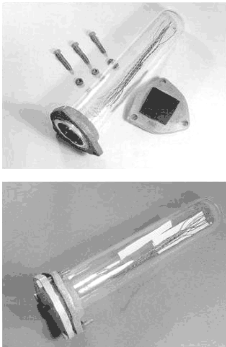
Рисунок 1 — Испытательная аппаратура
