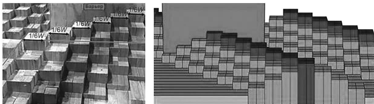
Рисунок 6 — Вид симметричной ступенчатой поверхности
