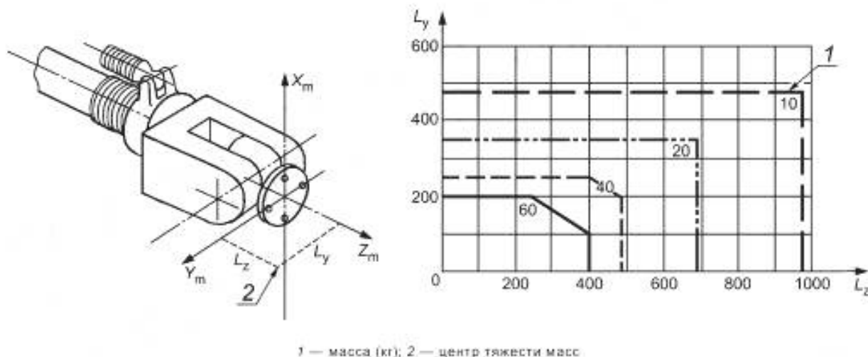
Рисунок 3 — Схема распределения нагрузок
