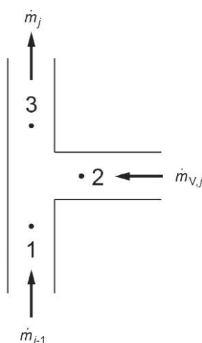
Рисунок 2 — Пример обозначения и нумерации для узловых точек [см. формулы (8) и (9)]
