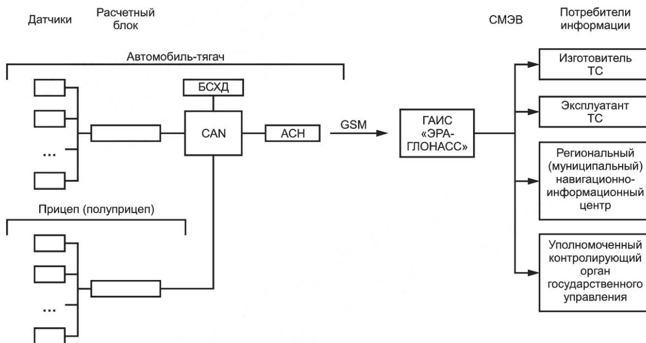
Рисунок 1 — Архитектура СМОН
