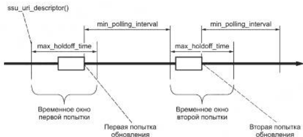
Рисунок 4 — Соотношение max_holdoff_time и min_polling_interval
