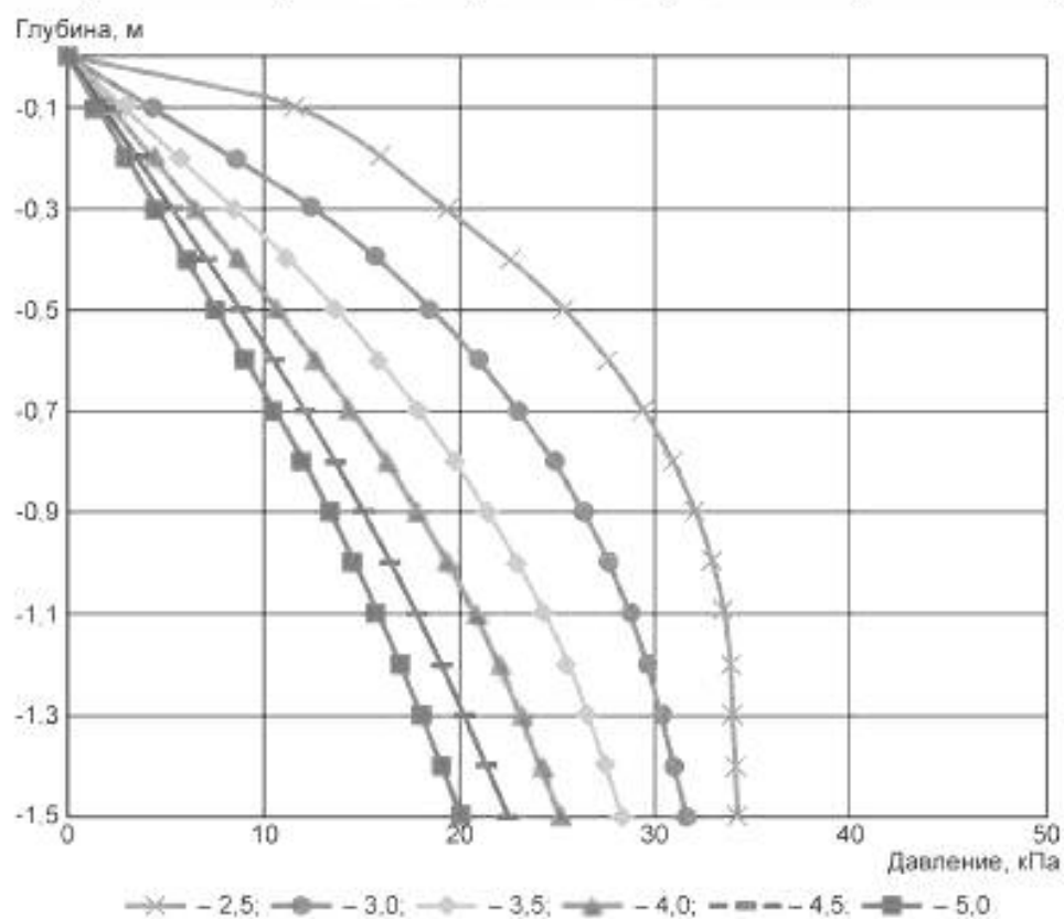
Рисунок Б.2 — Суммарное горизонтальное давление
