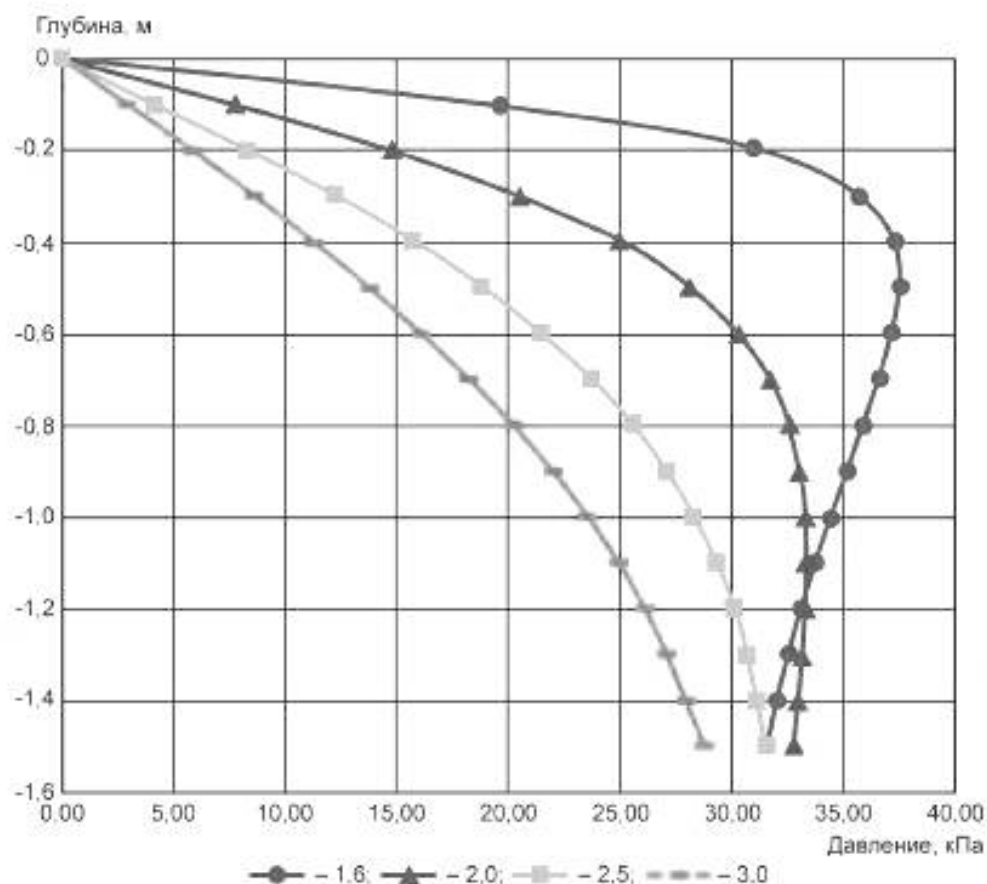
Рисунок Б.3 — Суммарное горизонтальное давление
