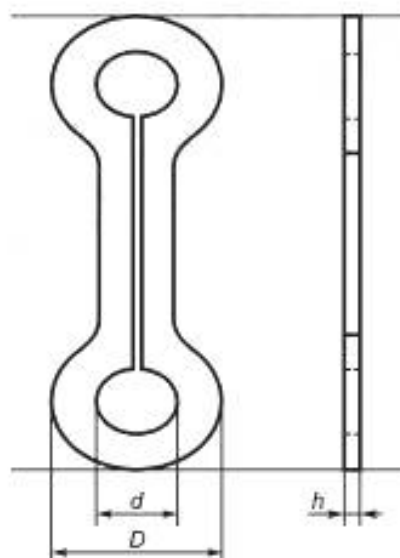
Рисунок 5 — Пластина обвода трубы
