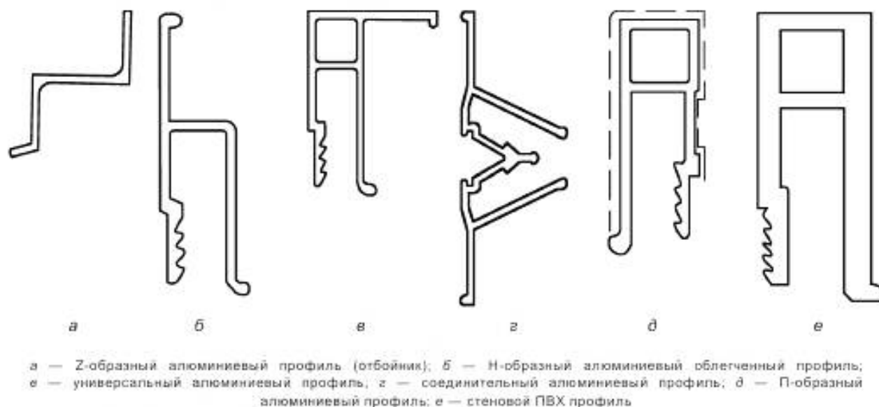
Рисунок 2 — Варианты исполнения крепежных профилей
