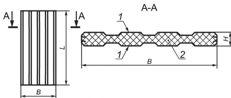
Рисунок 2 — Трехслойная панель
