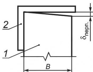
1 — панель; 2 — поверочный угольник 90°; B — ширина панели
