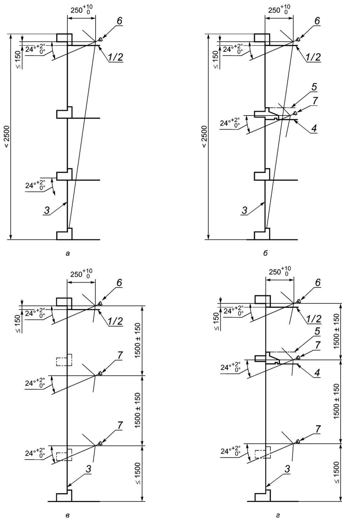
1, 4, 5 — линия, выше которой должны находиться сопла форсунок; 2 — линия стыковки рамы и створки; 3 — орошаемая поверхность; 6 — линия форсунок с суммарным расходом ( 2 \pm 0,2 ) л/мин — на каждую форсунку; 7 — линия форсунок с суммарным расходом ( 1 \pm 0,1 ) л/мин — на каждую форсунку
