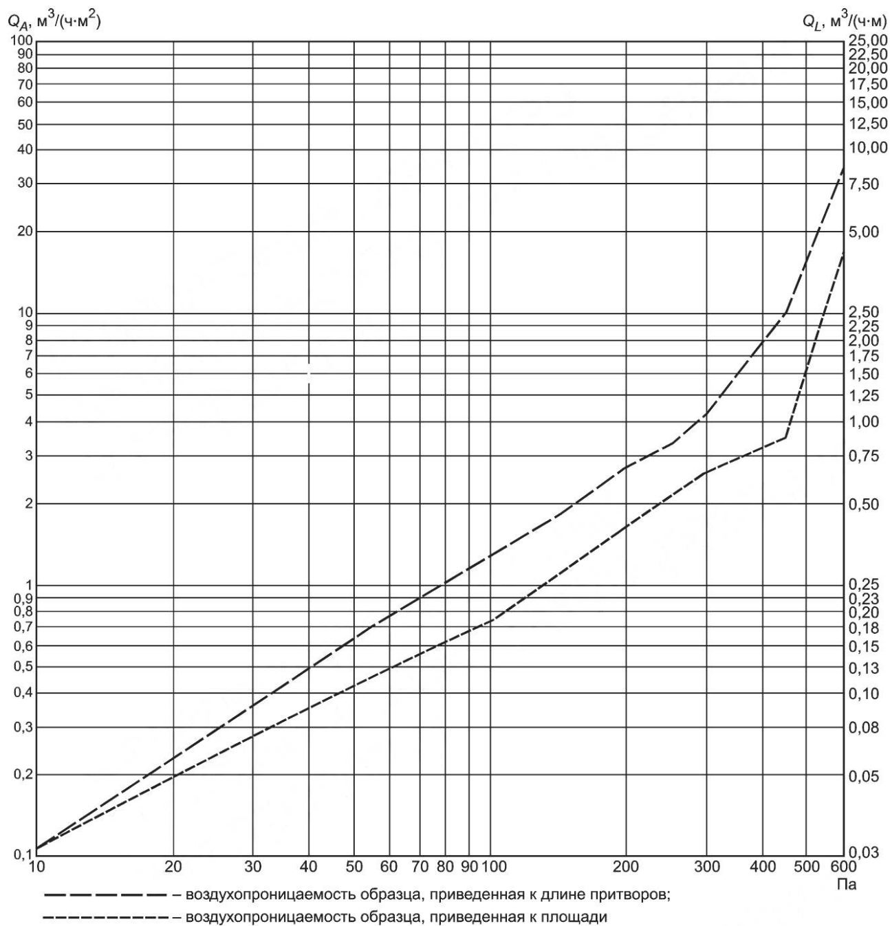
Рисунок 4 — Пример выполнения графика воздухопроницаемости испытуемого образца
