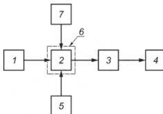
Рисунок 7 — Структурная схема рабочего места, установки (стенда) для проведения измерений импульсной вольтовой (токовой) чувствительности ФЭП и ФПУ на импульсном потоке
