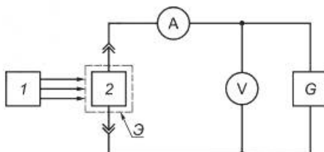
1 — источник излучения; 2 — испытываемый образец; Э — светозащитный экран; А — измеритель тока; V — измеритель напряжения; G — источник питания
