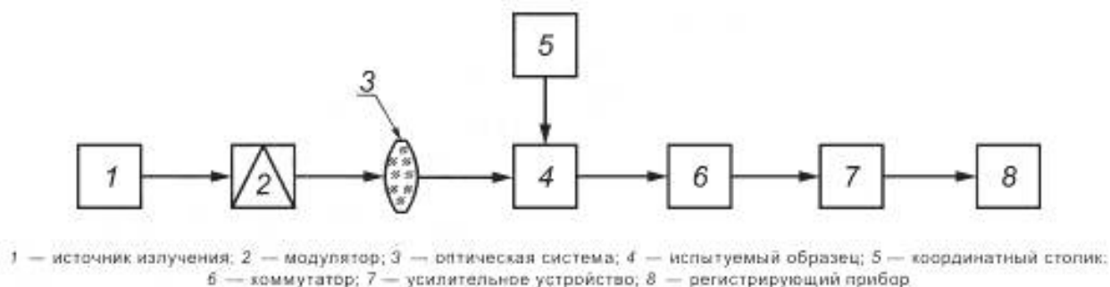
Рисунок 11 — Структурная схема рабочего места, установки (стенда) для проведения измерений коэффициента фотоэлектрической связи многоэлементных ФЭПП и ФПУ
