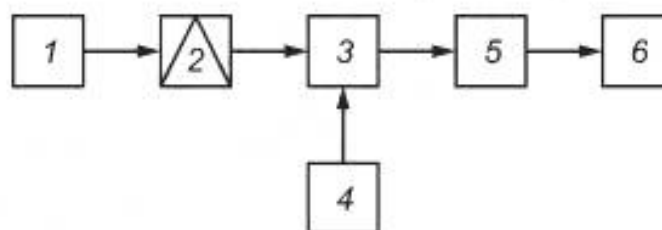
Рисунок 14 — Структурная схема рабочего места, установки (стенда) для проведения измерений частотных характеристик ФЭПП и ФПУ
