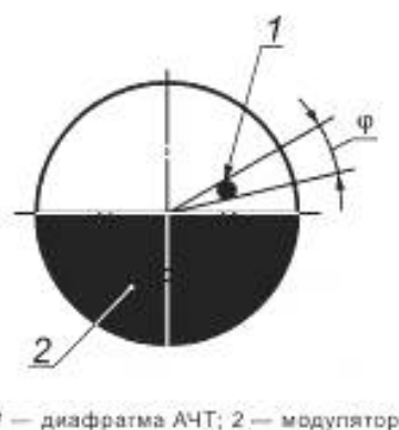
Рисунок 18 — Схема вращения диска модулятора
