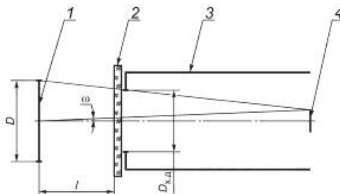
1 — диафрагма АЧТ диаметром D ; 2 — входное окно испытуемого образца; 3 — холодная диафрагма испытуемого образца диаметром D_{х.д.} ; 4 — центральная зона ФЧЗ ФПУ
