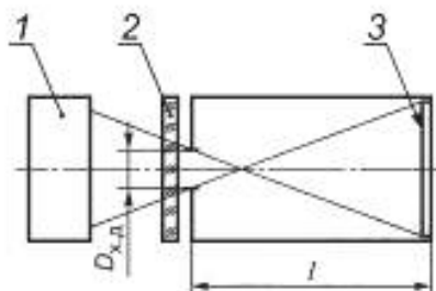
1 — излучающая поверхность АЧТ; 2 — входное окно ФПУ; 3 — плоскость ФЧЗ
