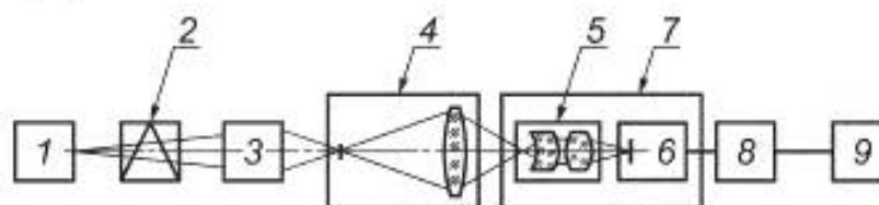
1 — источник излучения; 2 — модулятор/заслонка; 3 — конденсор; 4 — измеряемый оптический зонд с диафрагмой; 5 — проекционный объектив; 6 — матричное ФПУ; 7 — координатный стол; 8 — БЗО; 9 — ПК со специализированным ПО
