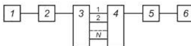
1 — генератор; 2 — согласующий усилитель; 3 — коммутатор; 4 — БЭО; 5 — ПК; 6 — ПО
