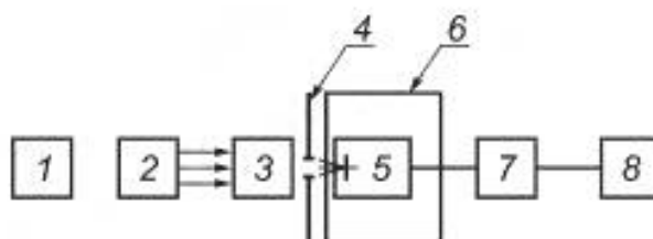
1 — микроскоп; 2 — источник излучения; 3 — заслонка; 4 — маска (устанавливается вплотную к плоскости ФЧЗ ФПУ); 5 — испытуемый образец; 6 — криостатируемый столик (может отсутствовать); 7 — БЗО; 8 — ПК со специализированным ПО
