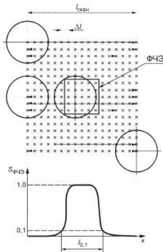
Рисунок 10 — Схема сканирования ФЧЭ ФПУ
