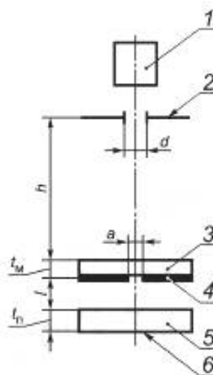
1 — источник излучения; 2 — диафрагма; 3 — маска; 4 — непрозрачный рисунок; 5 — подложка; 6 — плоскость ФЧЗ
