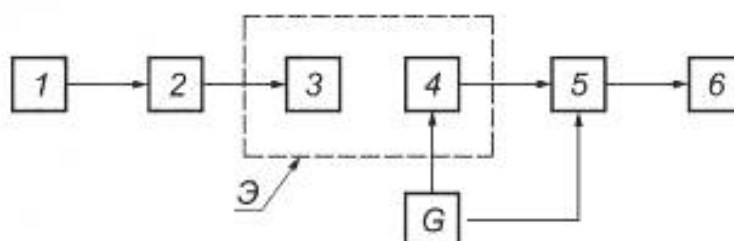
1 — светодиод; 2 — аттенюатор; 3 — конденсор (при необходимости); 4 — испытуемый образец; 5 — БЗО; 6 — ПК; G — источник питания; Э — светозащитный экран
