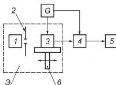
1 — источник излучения; 2 — набор сменных диафрагм; 3 — испытуемый образец; 4 — БЗО; 5 — ПК; 6 — система перемещения; G — источник питания; Э — светозащитный экран
