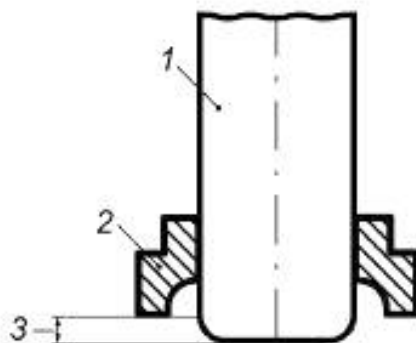
Рисунок 2 — Пример выступа
