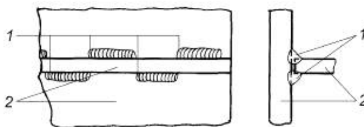
1 — шов; 2 — заготовка
