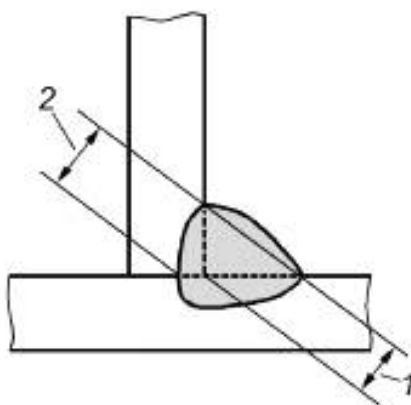
Рисунок 4 — Эффективная толщина углового шва
