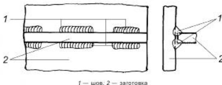
Рисунок 2 — Цепной прерывистый шов
