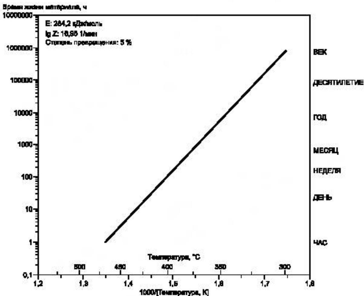
Рисунок 1 — Кривая термической устойчивости
