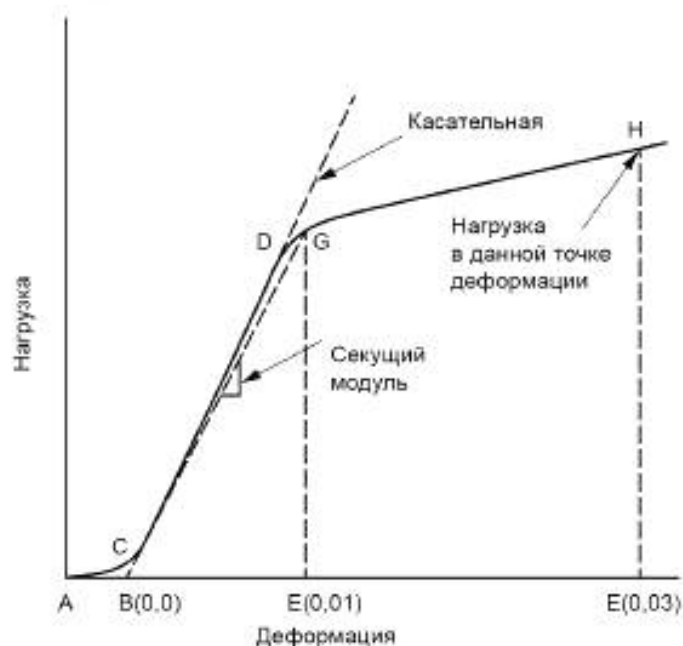
Рисунок Б.1 — График зависимости «нагрузка — деформация»
